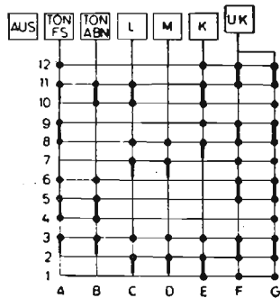
Schalterdiagramm
