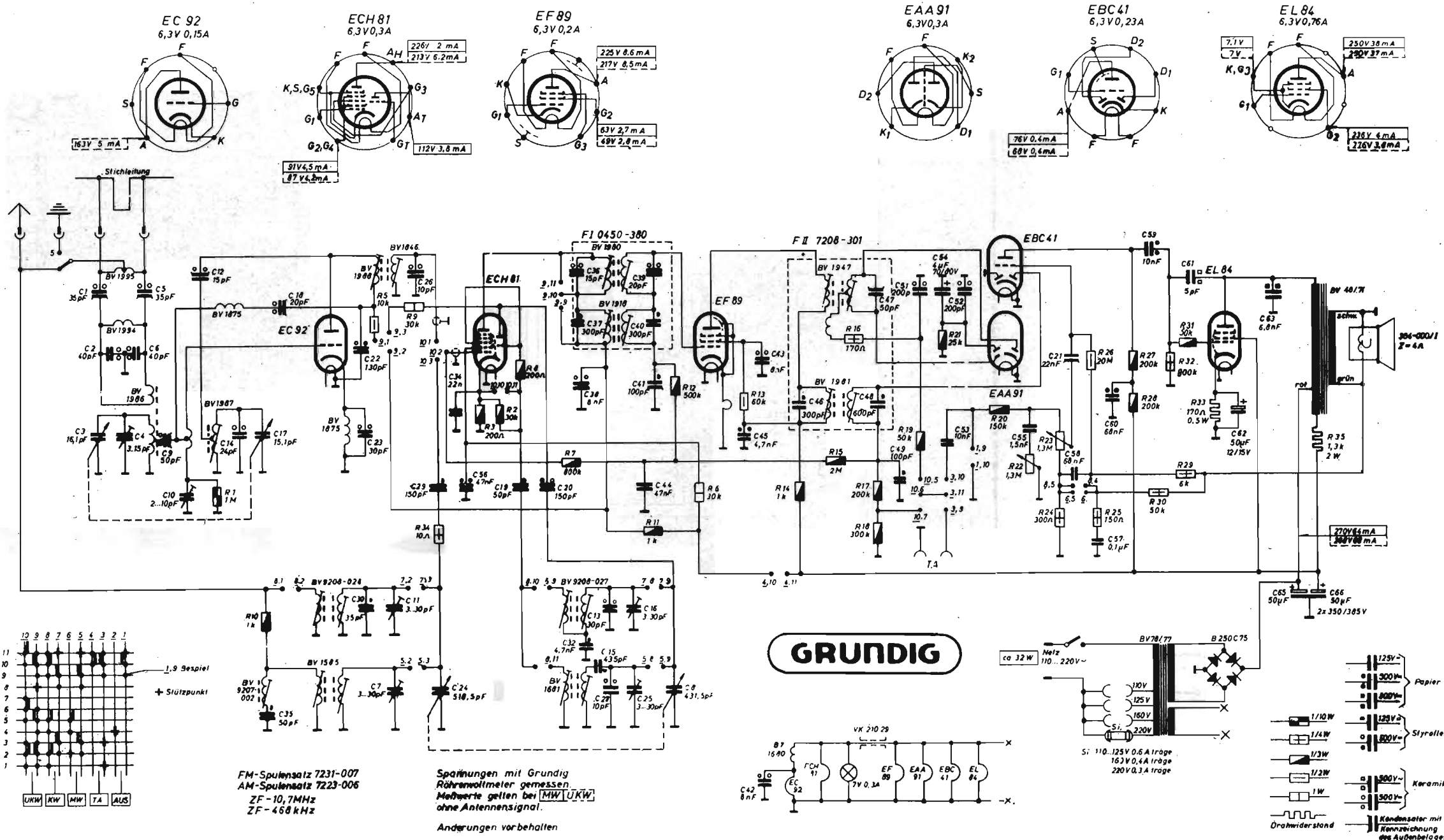
GRUNDIG (Radio Werke GmbH) - Mod. AM/FM Super-955 W/3D. A modulazione d'ampiezza e di frequenza, con una gamma onde medie da 510 a 1620 kc/s, una gamma onde corte da 5,9 a 15,8 Mc/s e una gamma onde ultracorte (FM) da 87 a 100 Mc/s. MF/AM a 468 kc/s e MF/FM a 10,7 Mc/s. Potenza d'uscita 4 watt.
