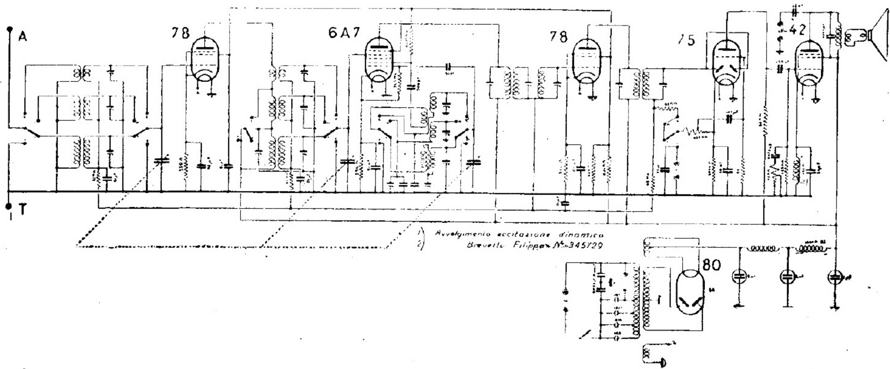
IMCARADIO - MOD. «IF 65»
