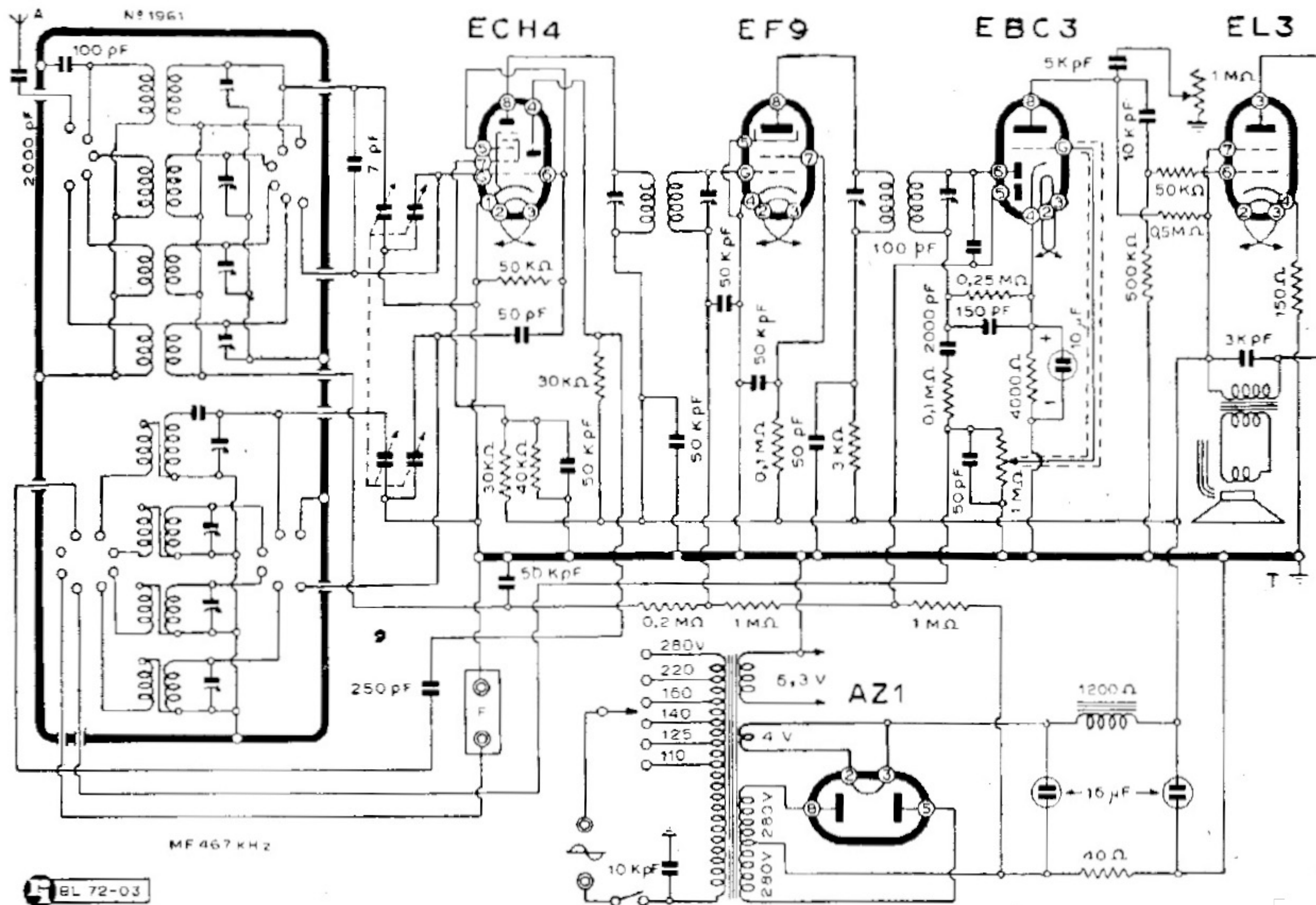
I.M.C.A.R. (GROSSETO) - MOD. « ROMA II »
