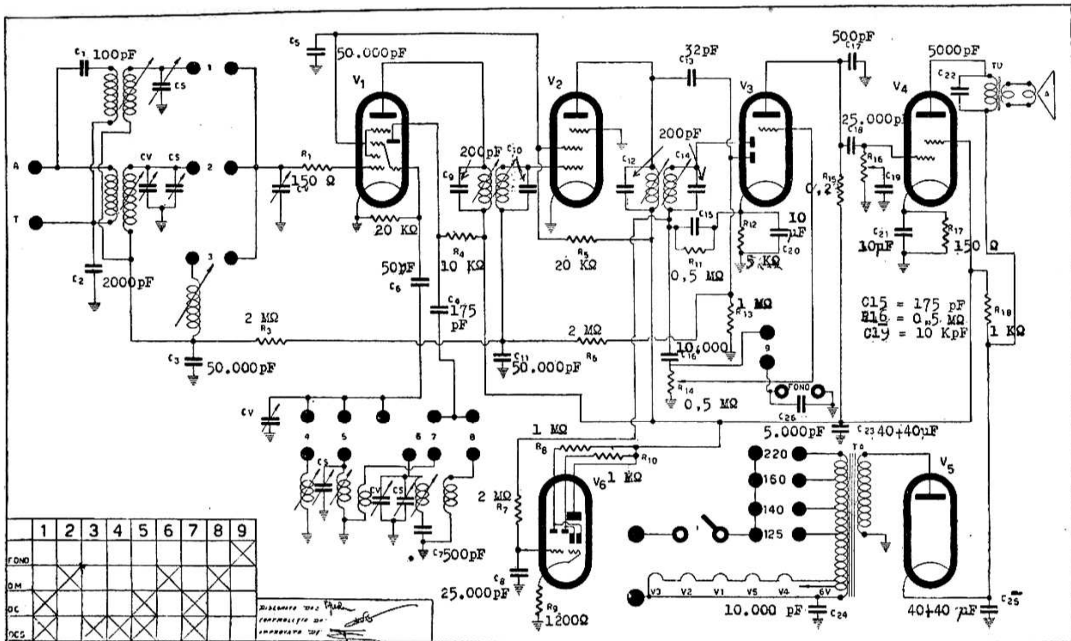
INCAR - Mod. VZ 519 - Tre gamme, onde medie e corte. Valvole: V_1 = \text{UCH41} , V_2 = \text{UAF41} , V_3 = \text{UAF41} , V_4 = \text{UL41} , V_5 = \text{UY41} , V_6 = \text{EM4} . Potenza d'uscita 2,5 watt indistorti.
