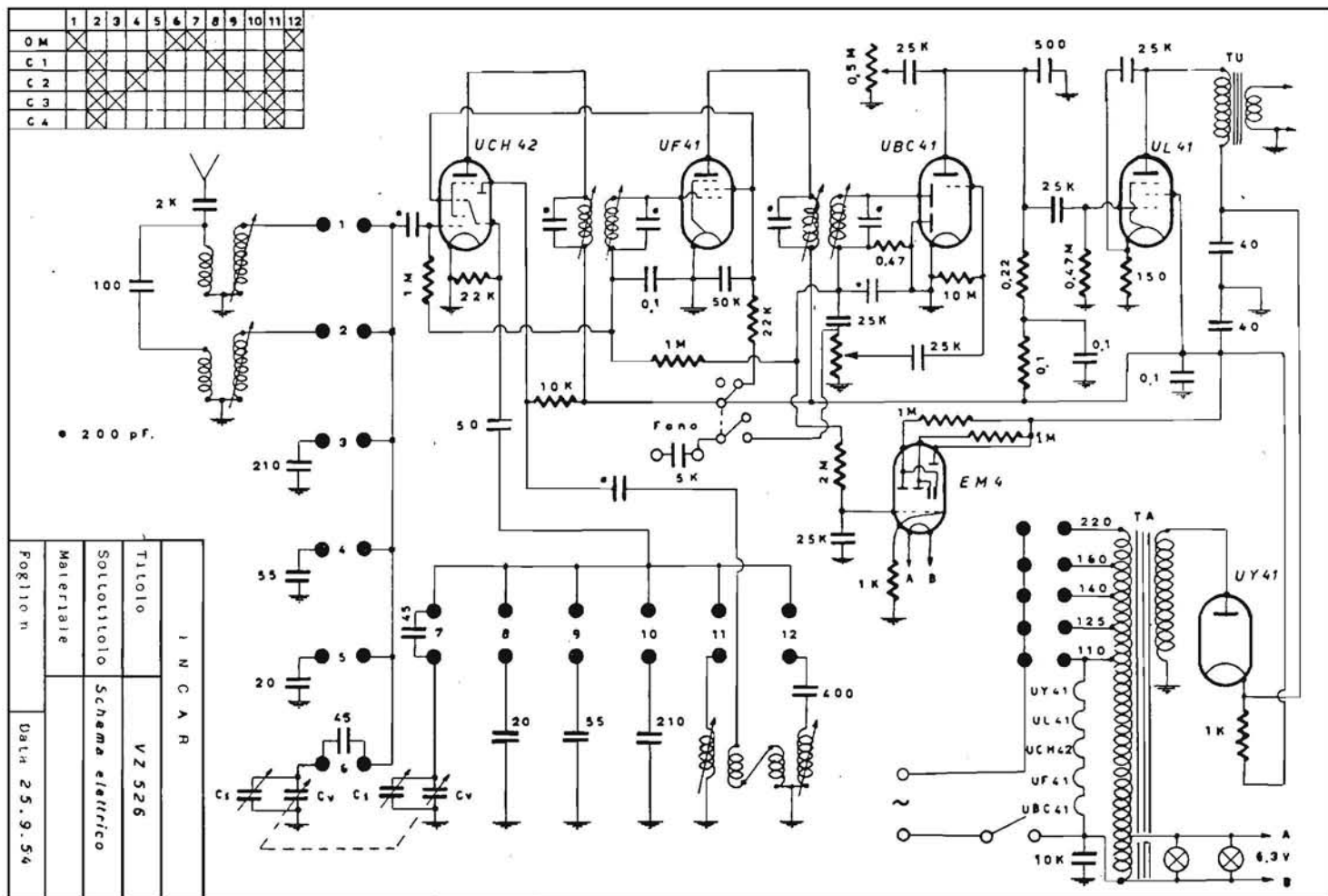
INCAR - Mod. VZ 526. Ricevitore a onde medie con quattro bande allargate ad onde corte. Potenza d'uscita 3 watt. Consumo 50 watt.
