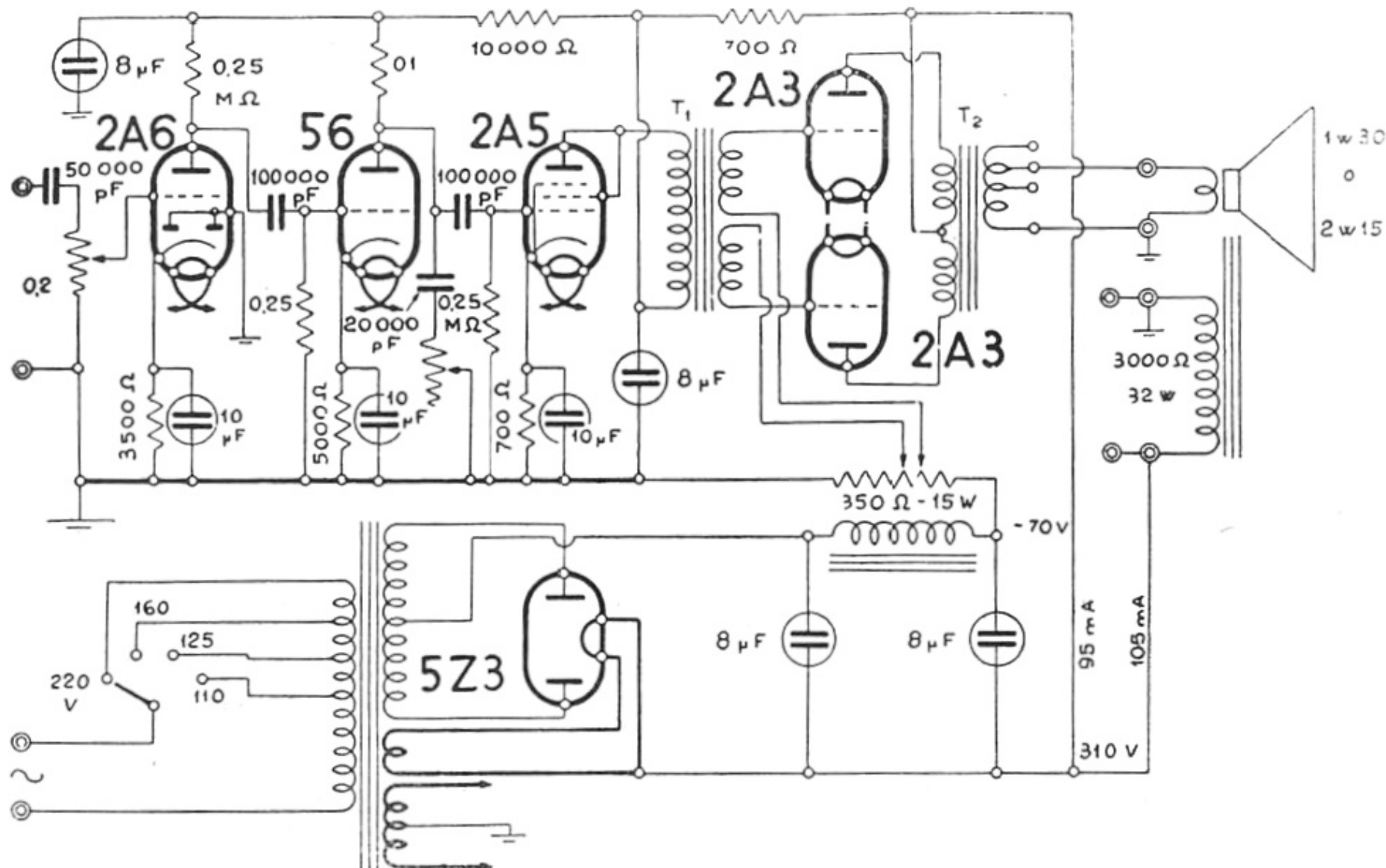
INDUSTRIALE RADIO - "AMPLIFICATORE IR 6 A 20"
