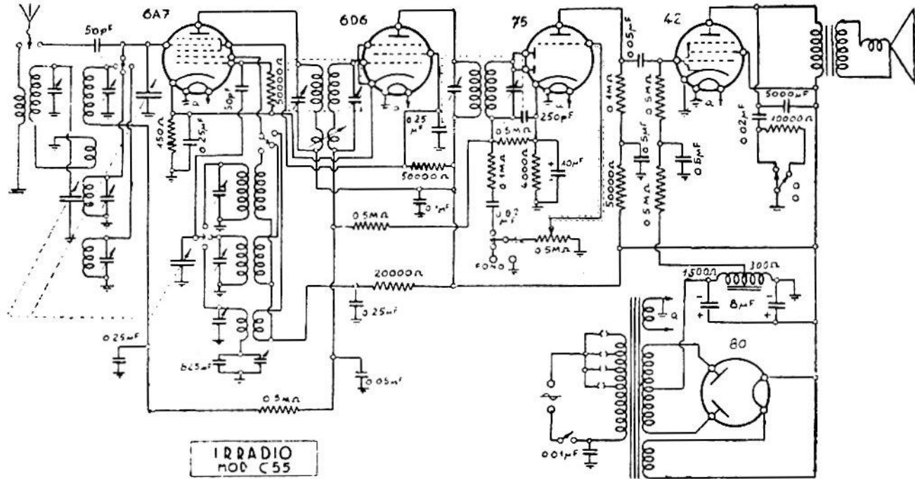
IRRADIO. — Mod. « C 55 ». — Super a 3 gamme d'onda. — Media frequenza: 250 kHz. — Produzione 1937.
