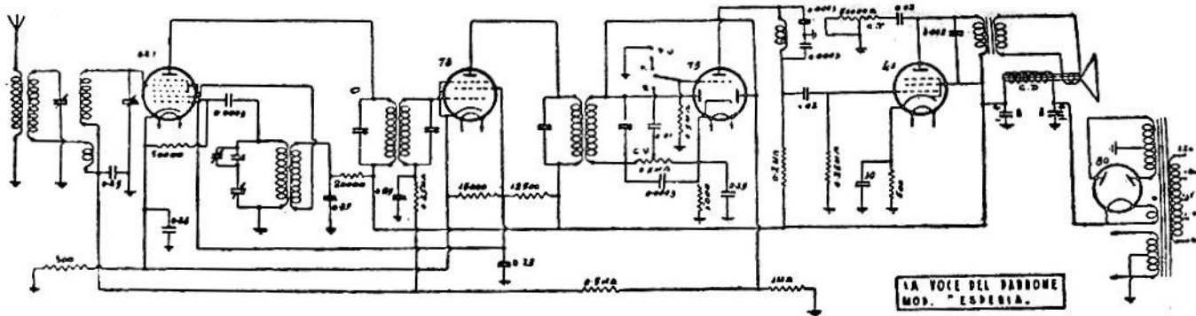
LA VOCE DEL PADRONE — Modello « Esperia ». - Produzione 1934 Media frequenza: 175 kc.
