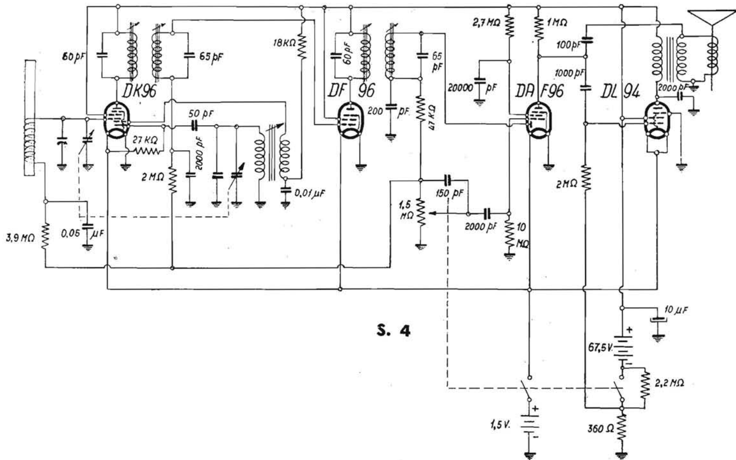
MAGNADYNE RADIO - Mod. S4. Portatile a pile. Gamma onde medie. Media frequenza 471 kc/s.
