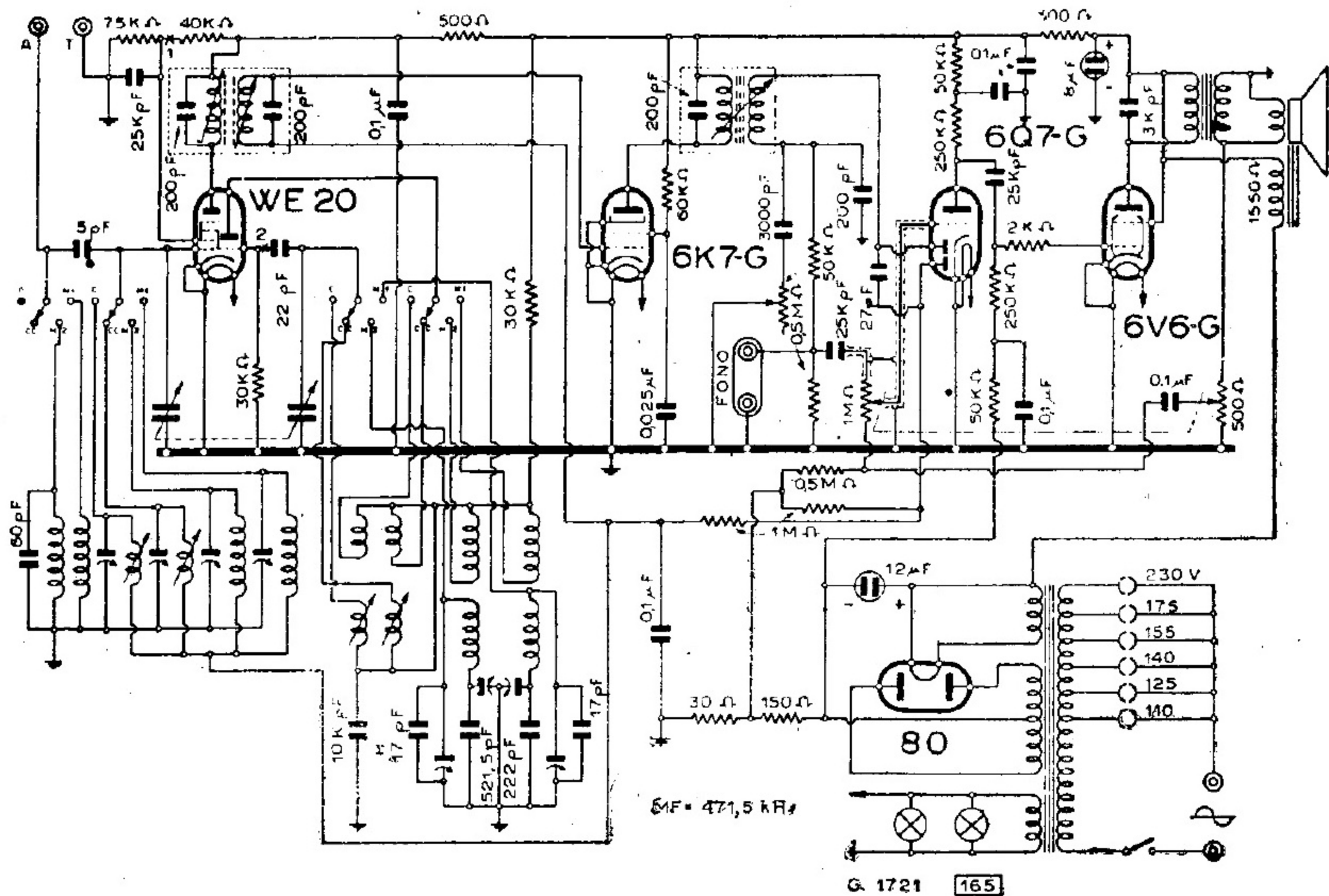
MAGNADYNE - MOD. « S 53 C »
