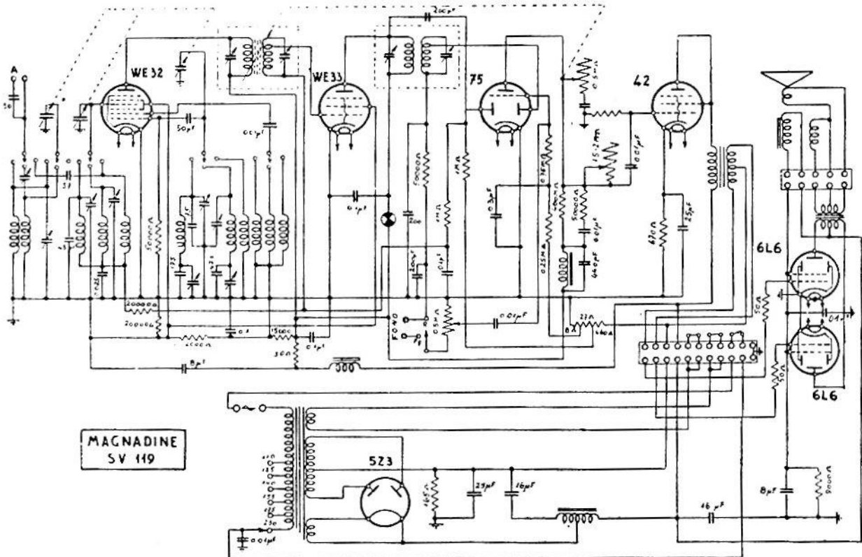
MAGNADINE RADIO. — Mod. SV 119. — Produzione 1938-39. — Media frequenza: 362.5 kHz.
