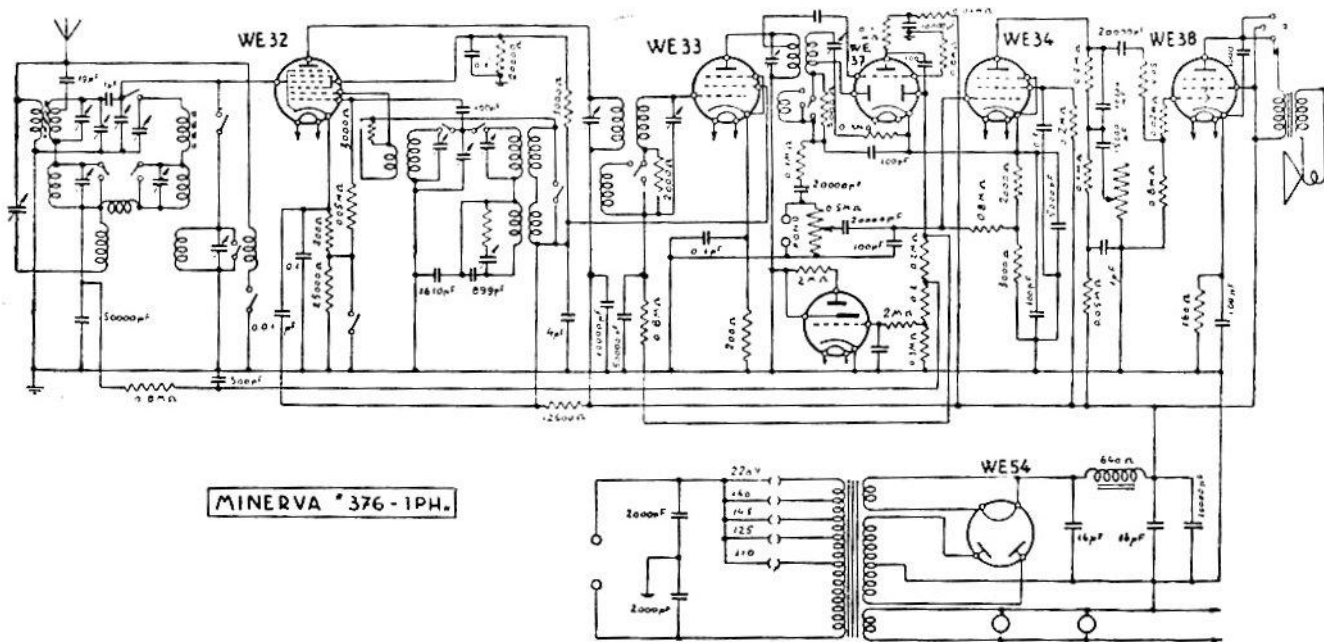
ITAL-MINERVA — Mod 376 1 PH. — Produzione 1938. — Media frequenza: 128 kHz.
