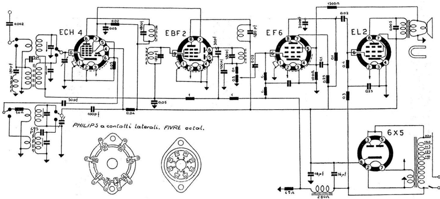
MINERVA RADIO - Mod. 455/1 - Due gamme di ricezione: da 195 a 580 m, e da 17 a 52 m. Media frequenza: 470 kc/s. Potenza d'uscita: 3 watt. Consumo: 30 watt. Altoparlante a magnete permanente. Produzione 1945-46.
