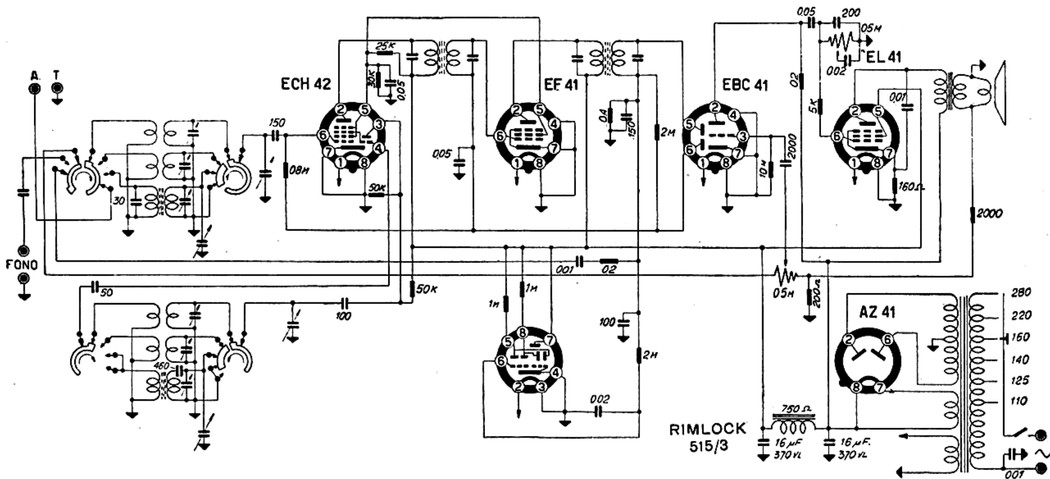
MINERVA RADIO - Mod. Rimlock 515/3 - Onde medie e due corte. Media frequenza a 488 kc. Esiste un mod. 515/3 con valvole di tipo americano. Resa d'uscita 3 watt. Consumo 55 watt.
