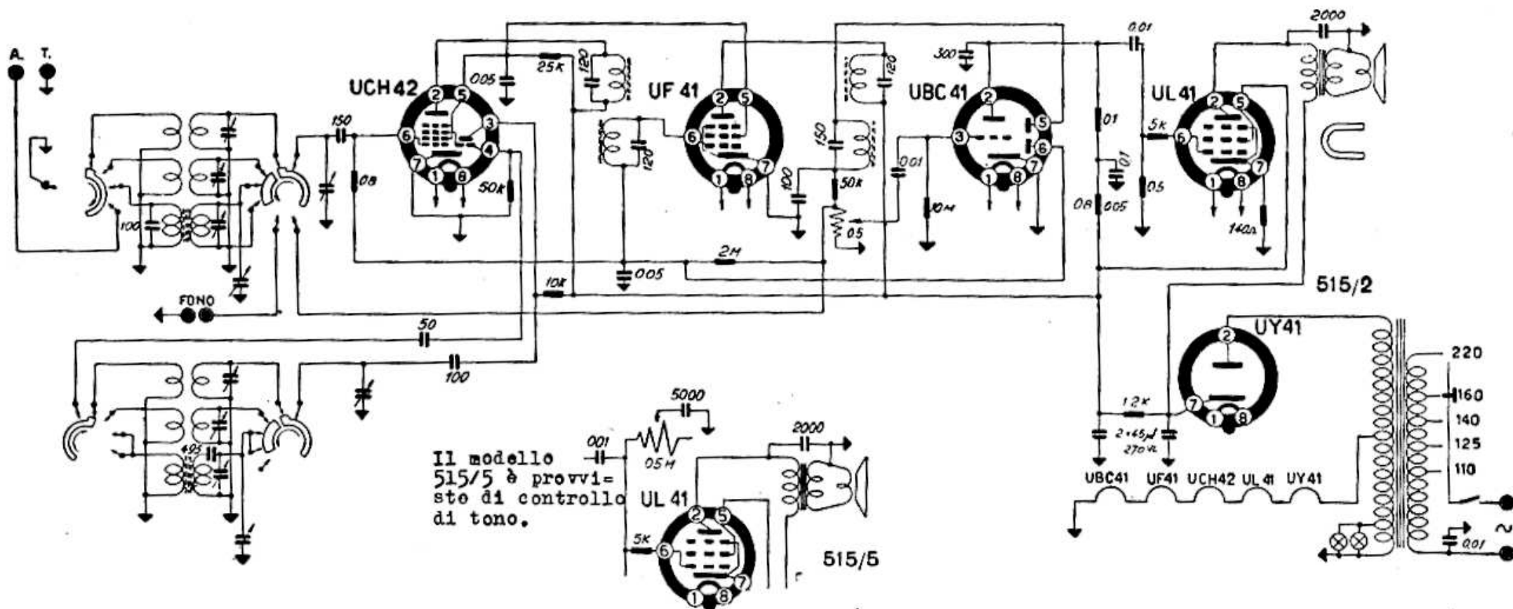
MINERVA RADIO - Modd. 515/2 RUBINO e 515/5 - Gamma onde medie e due gamme onde corte. Media frequenza a 468 kc. Resa d'uscita 2,5 watt. Consumo 35 watt.
