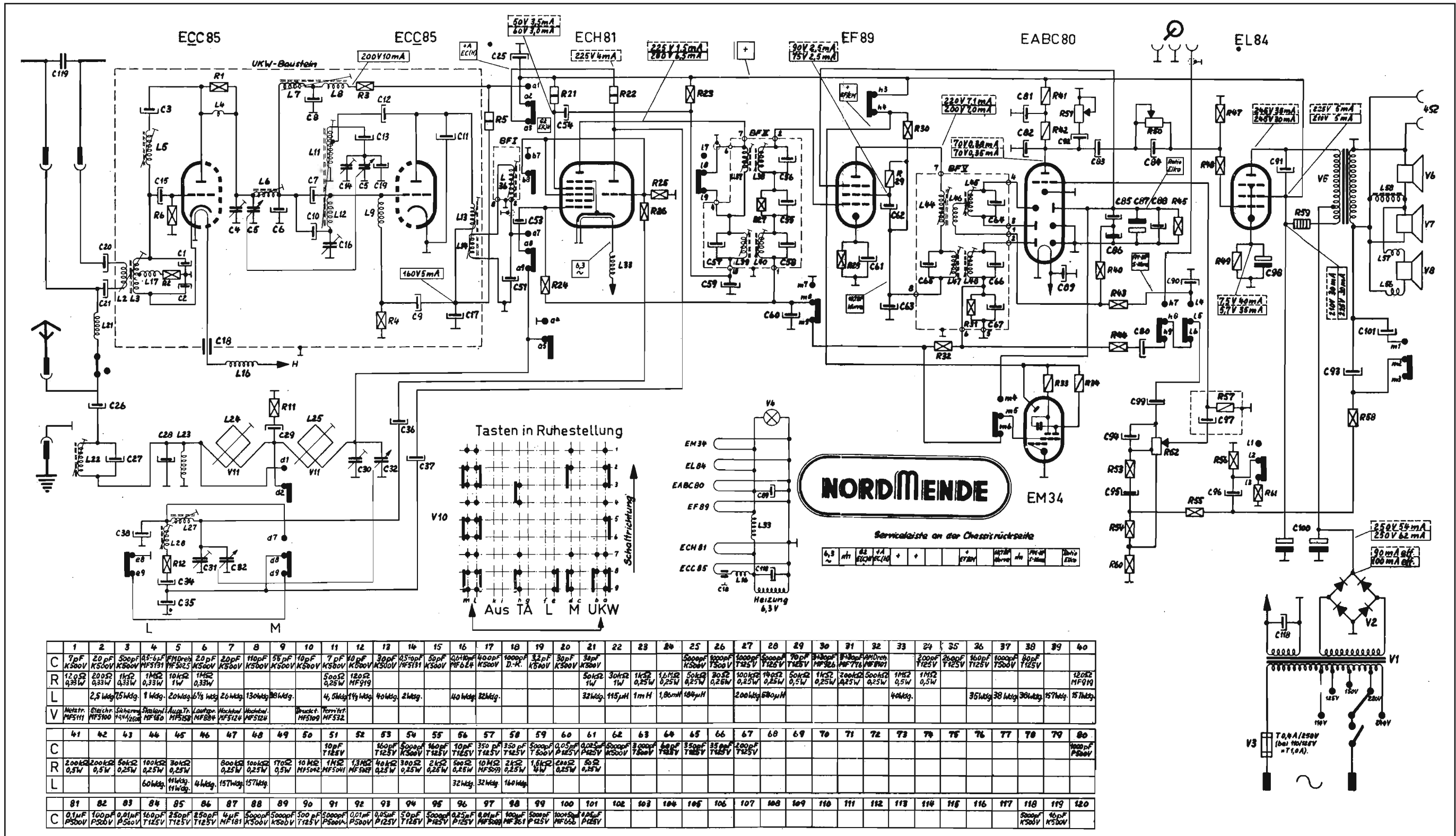
NORD MENDE (Norddeutsche Mende-Rundfunk, Bremen) - Mod. Elektra e Rigoletto 56. Apparecchi AM/FM. Lo schema è del Rigoletto 56, il mod. Elektra differisce per avere un solo altoparlante. Onde medie e corte in AM, a onde ultracorte in FM. Media frequenza AM a 460 kc/s, FM a 10,7 Mc/s. Potenza indistorta d'uscita 5 watt.
