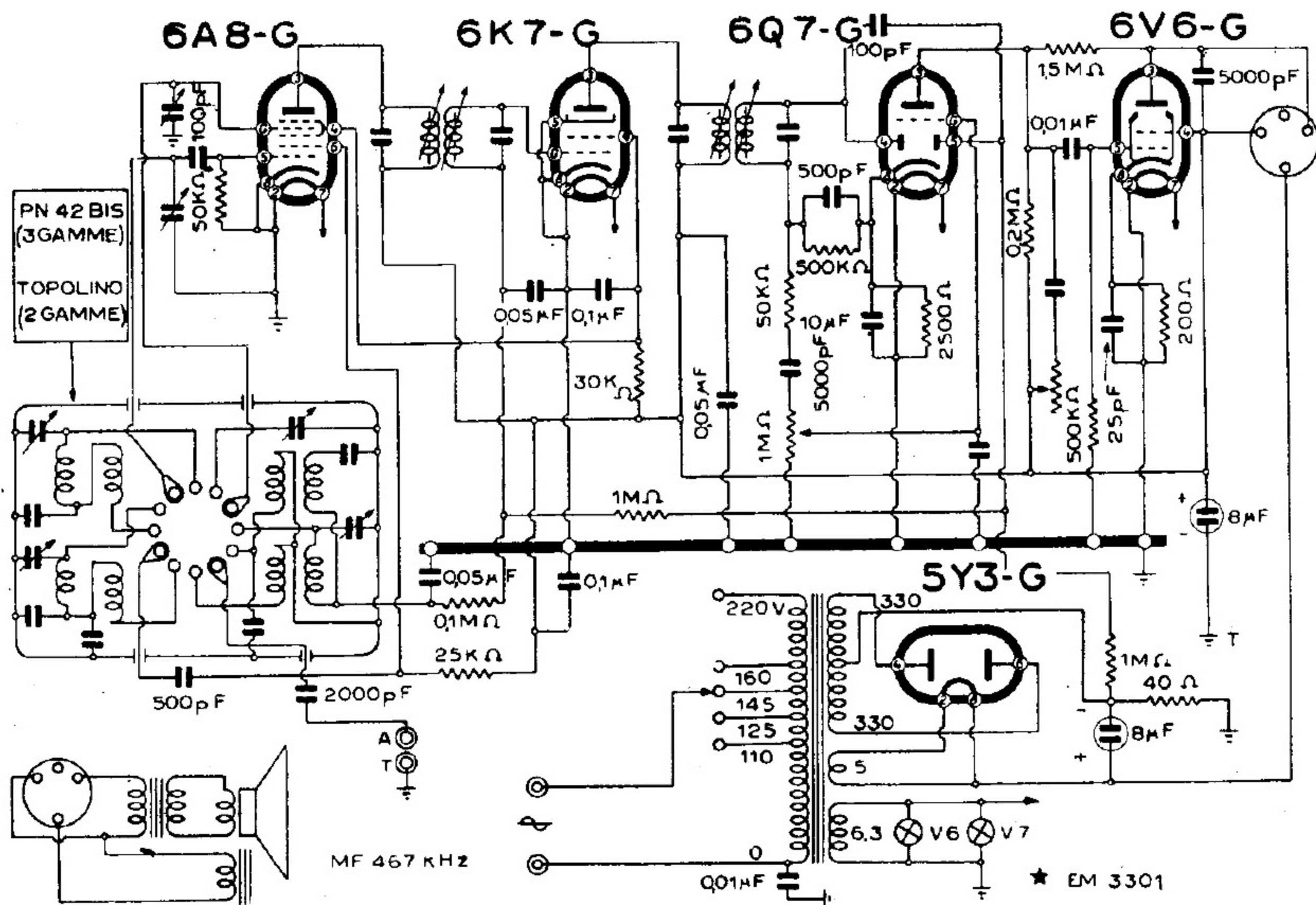
OMEGA RADIO - MODD. « PN 42 bis » « TOPOLINO »
