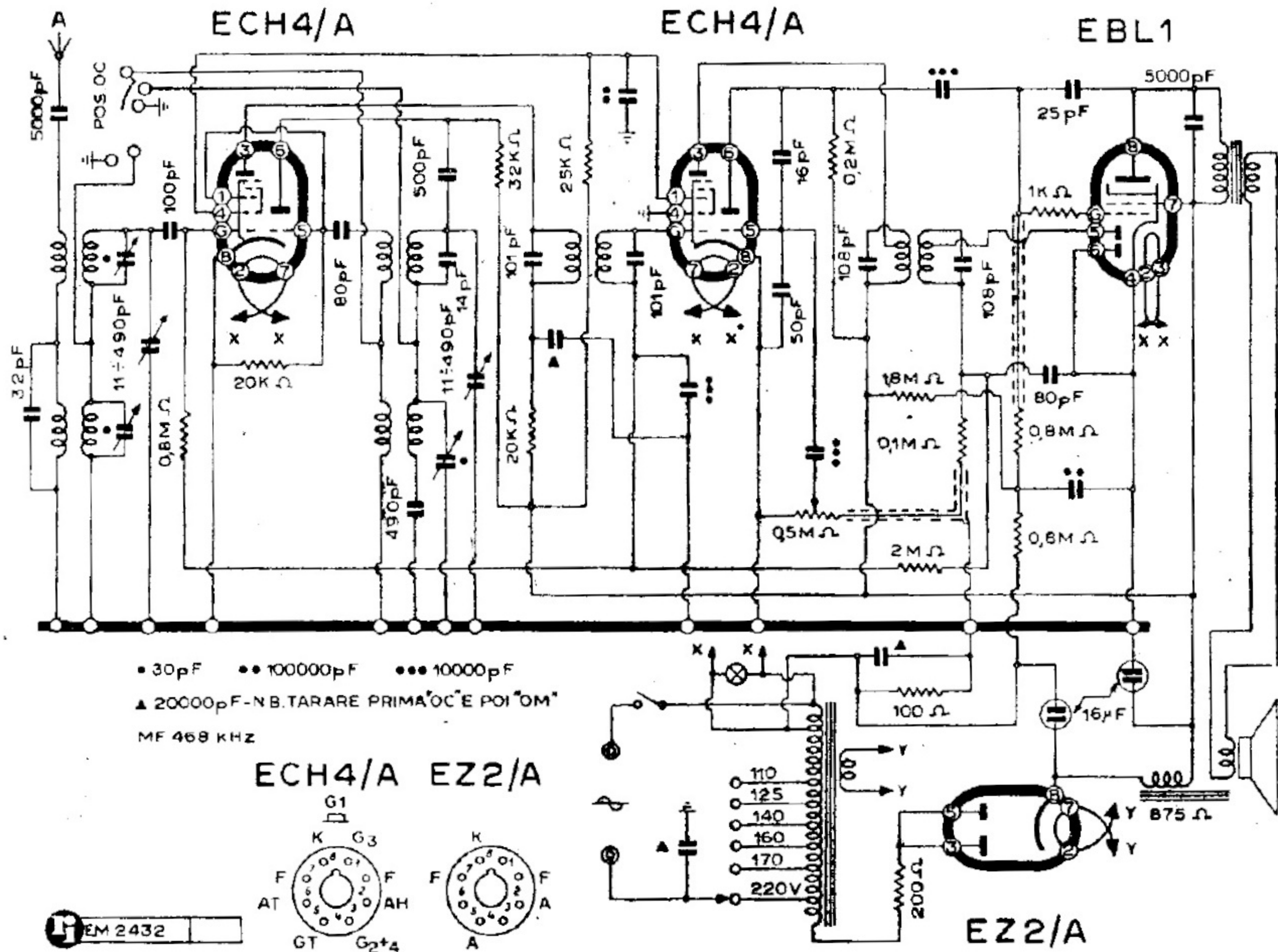
PHILIPS RADIO - MOD. « BI 270 A »
