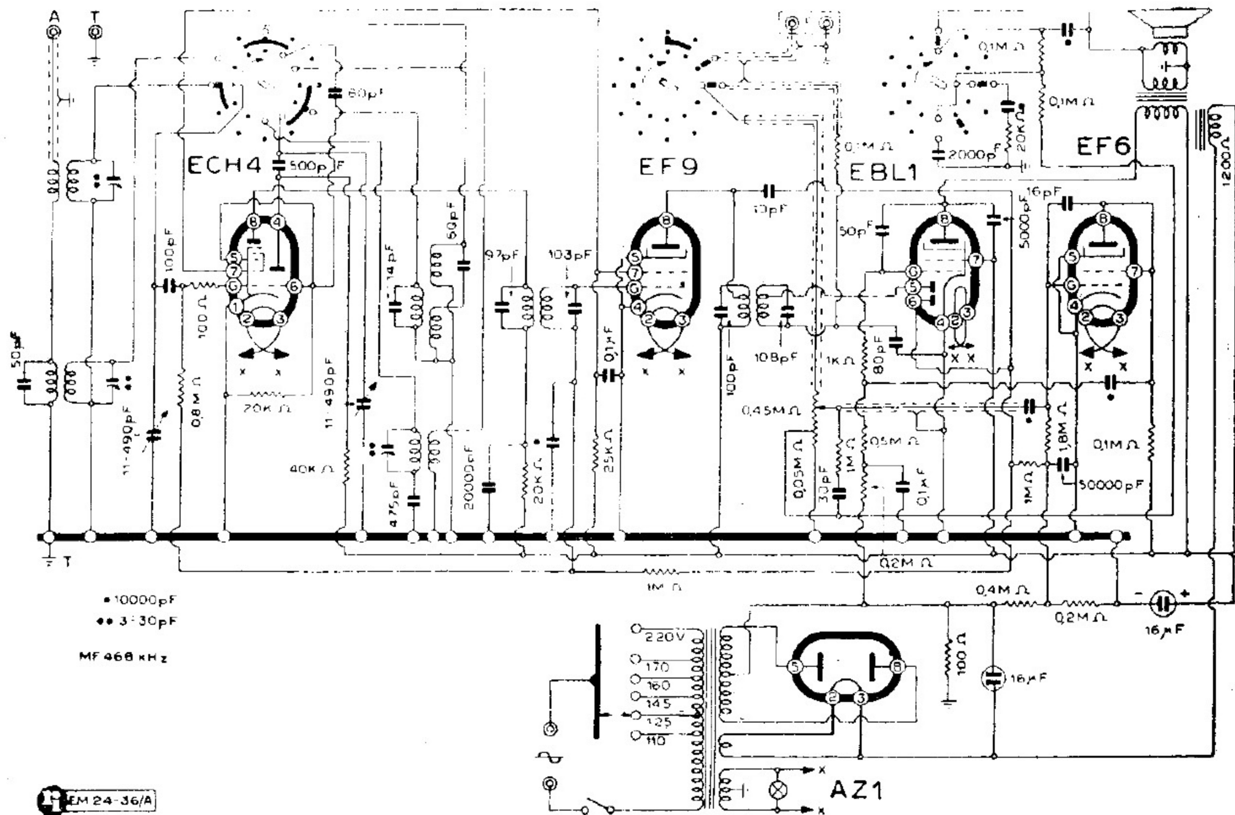
PHILIPS RADIO - MODD. « BI 480/A » « BI 481/A »
