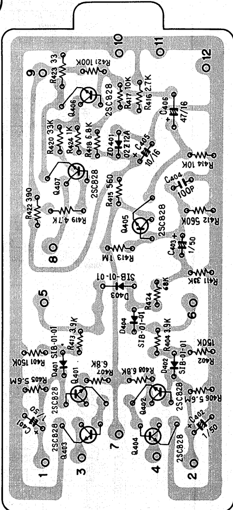
Limiter ass'y RWX-071
