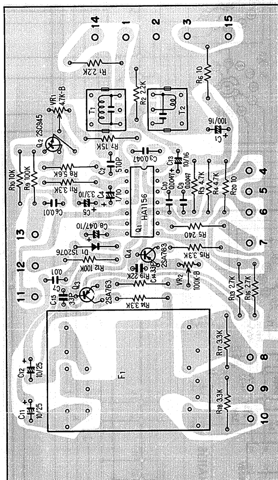
MPX ass'y AWD-005
