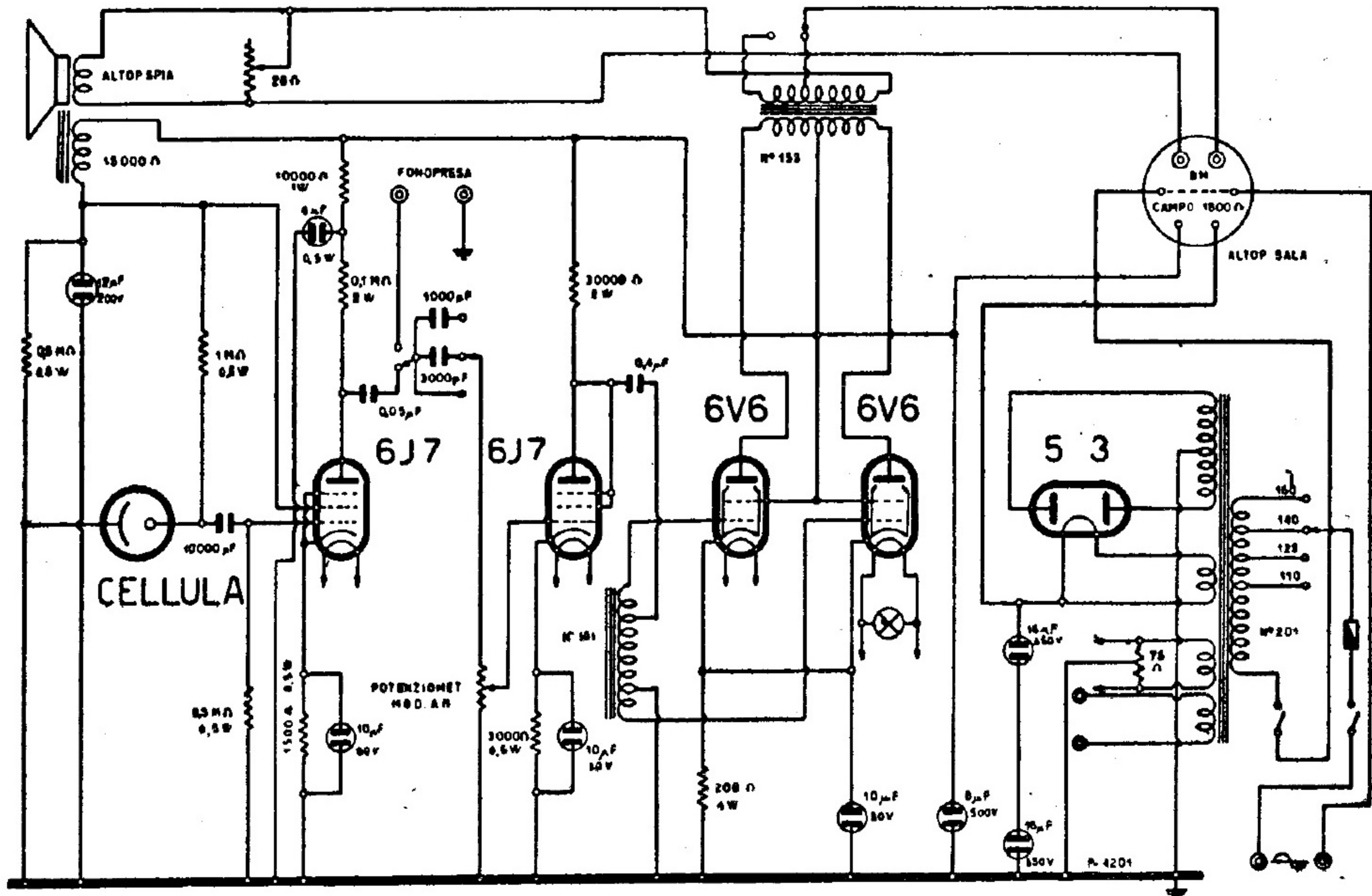
PREVOST ING. A. - AMPLIFICATORE MOD. « 121 - I Serie »
