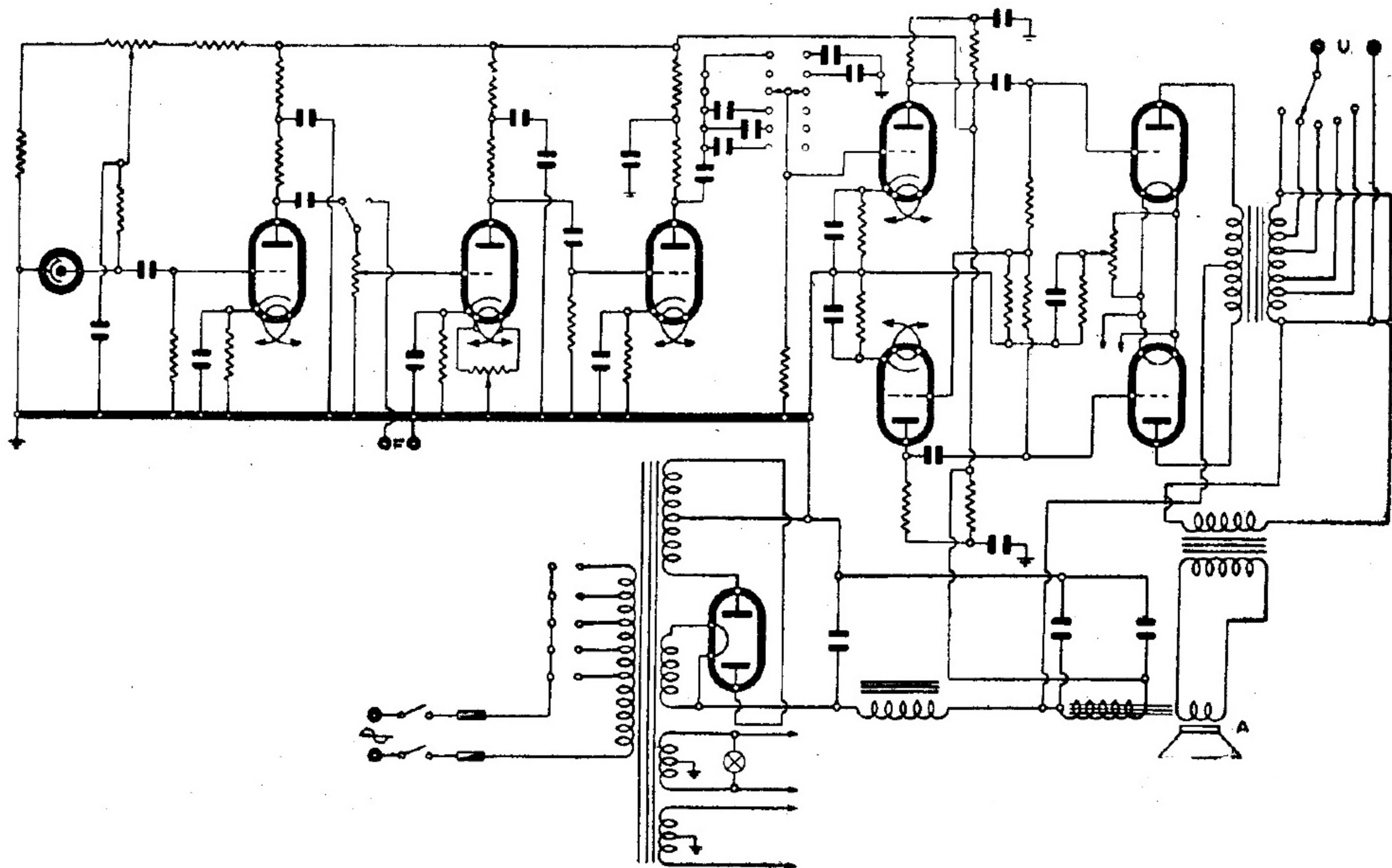
PREVOST ING. A. - AMPLIFICATORE MOD. « 301 »
