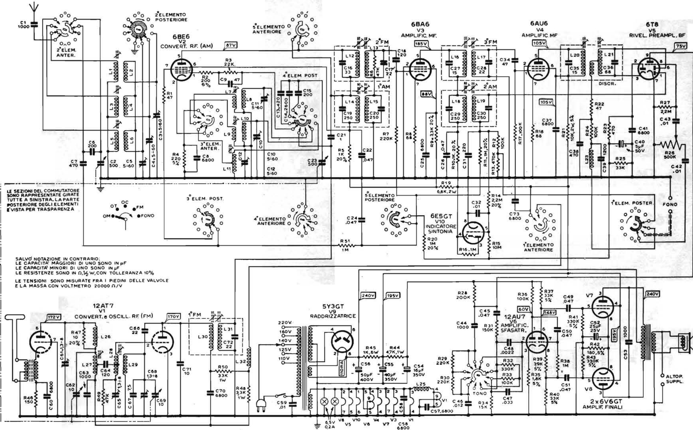
RADIO MARELLI - Apparecchio AM/FM mod. 157. Medie da 515 a 1640 kc/s, tropicali da 3200 a 10100 kc/s, corte da 11200 a 18700 kc/s, modulazione di frequenza da 87,3 a 100,5 Mc/s. MF/AM a 455 kc/s, MF/FM a 10,7 Mc/s. Potenza d'uscita 7 W, consumo 78 W. (Per allineamento e taratura v. istruzioni modd. 159, 163 e 164).
