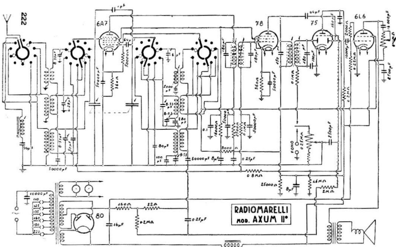
RADIO MARELLI — Modello « Axum II mobile e sopramobile ». — Produzione 1937. — Media frequenza: 450 kHz.
