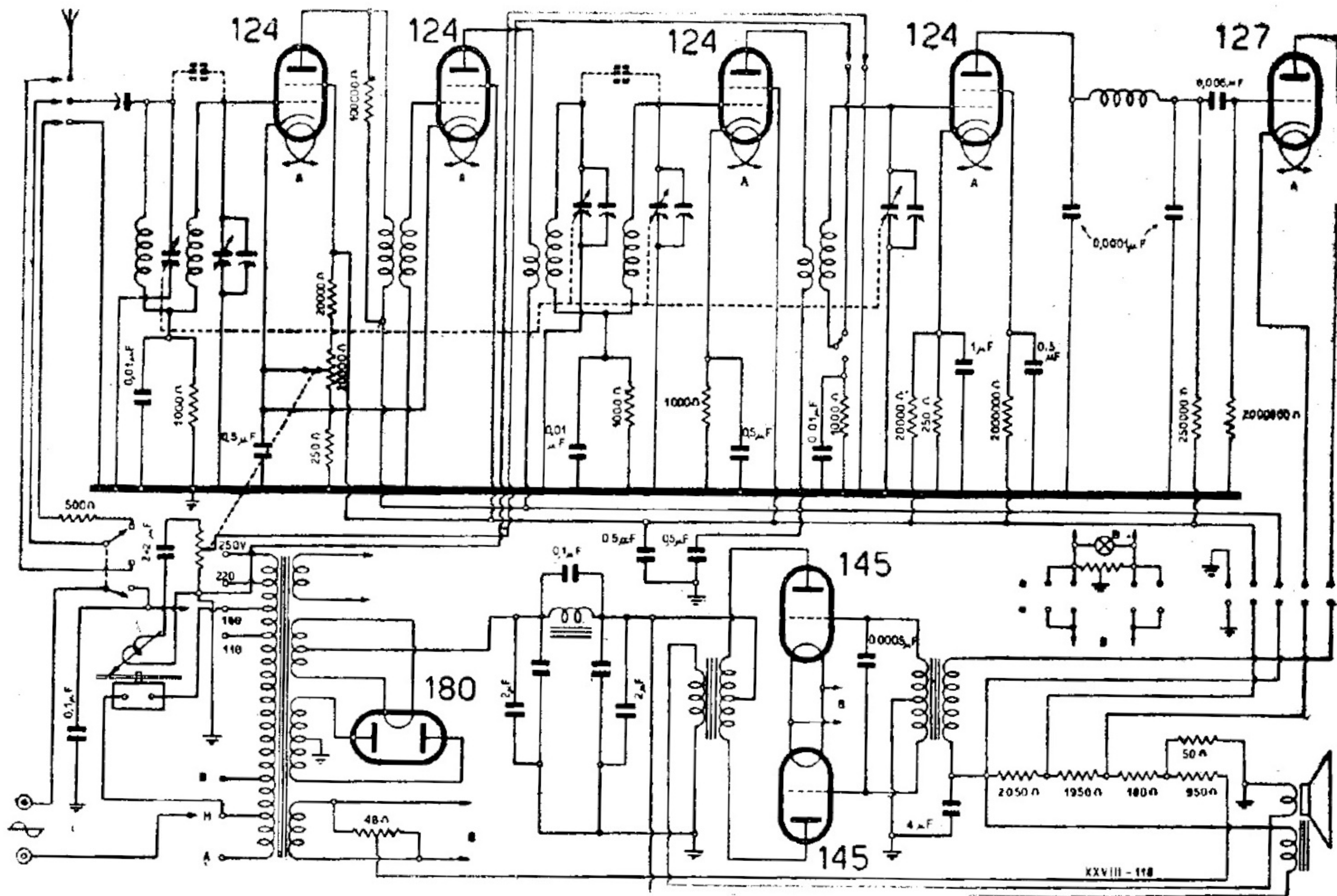
RADIOMARELLI - MOD. « CHILIOFONO I »
