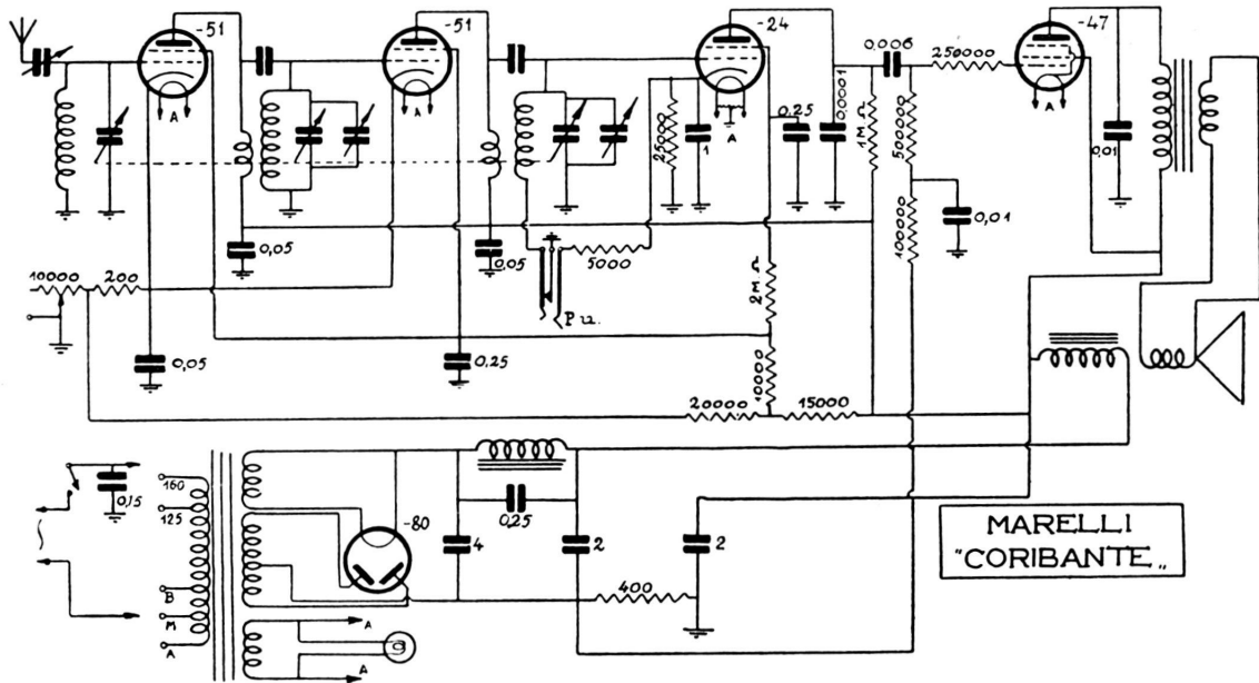
Onde medie. - Amplificazione diretta in a. f. con due schermate multi mu 51. - Rivelazione con 24. - Amplificazione finale con 47. - Potenza d'uscita: 2,5 watt.
