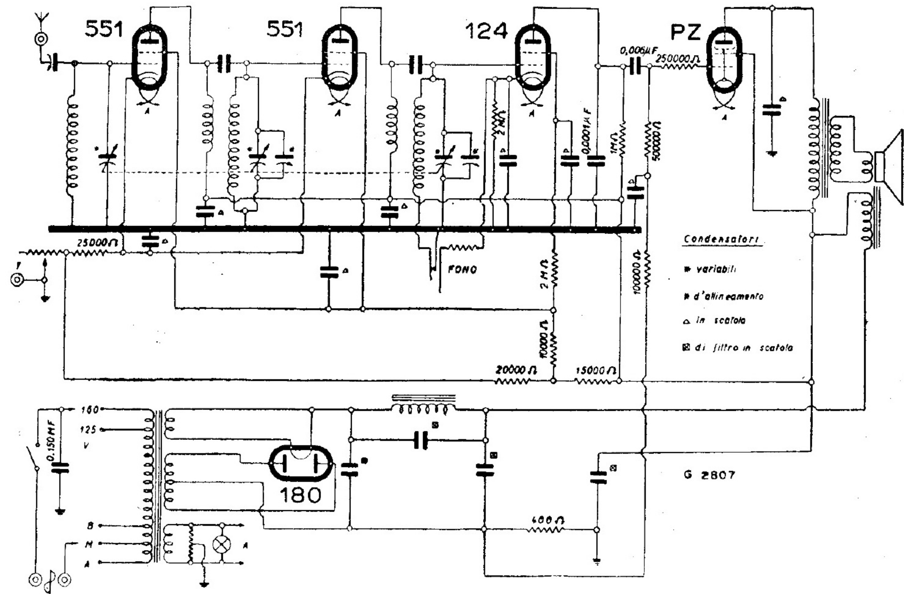
RADIOMARELLI - MOD. « CORIBANTE »
