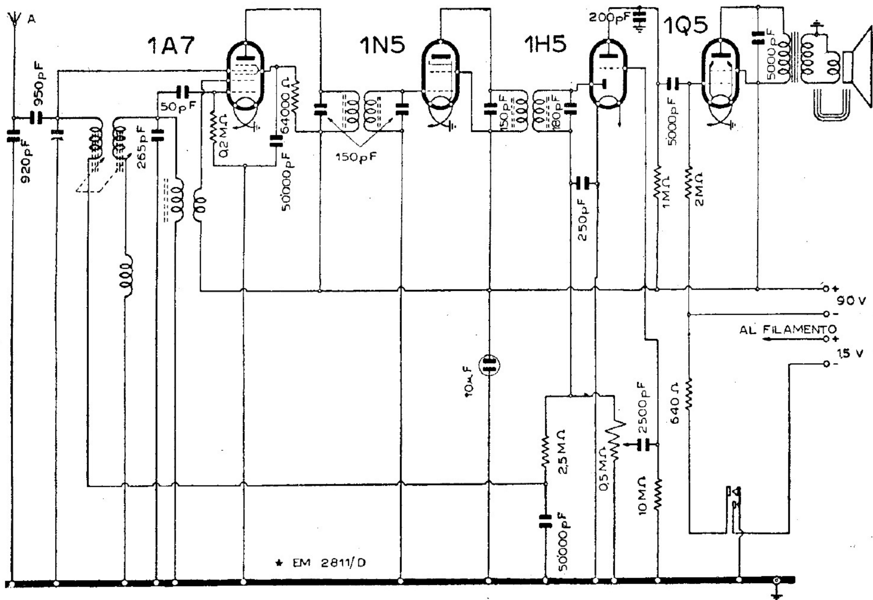
RADIOMARELLI - MOD. « FIDO A PILE »
