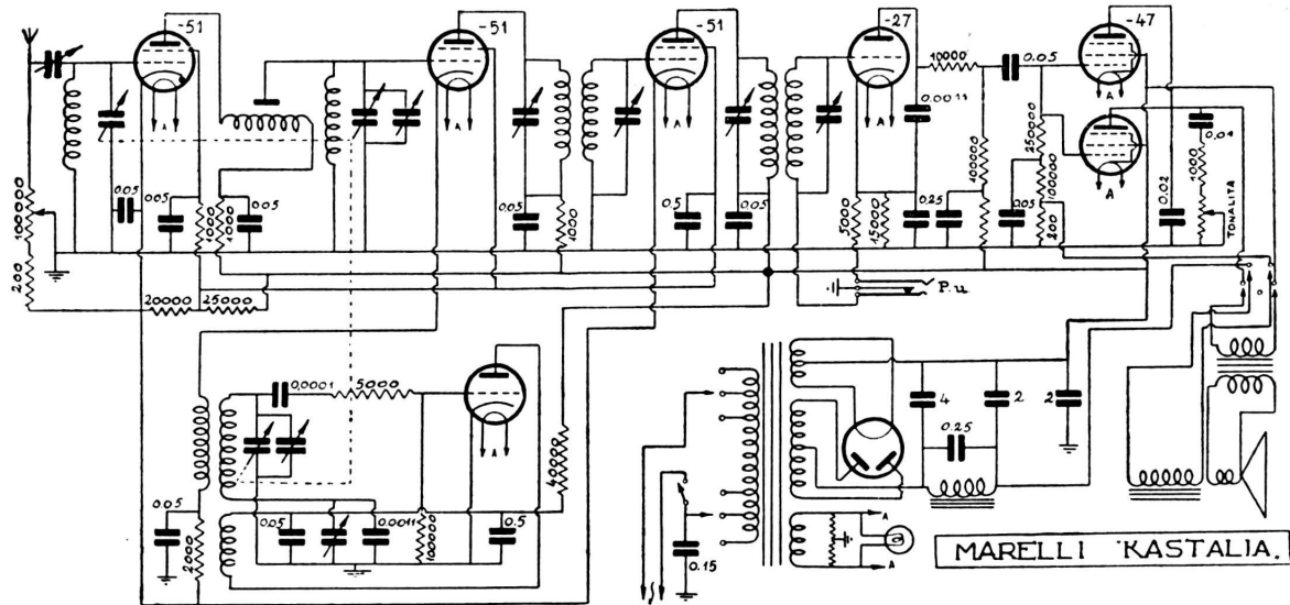
Onde medie. - M. F. 485 kc. - Oscillatrice 56 separata. - Due pentodi 47 in parallelo. - Potenza d'uscita 3,5 watt.
