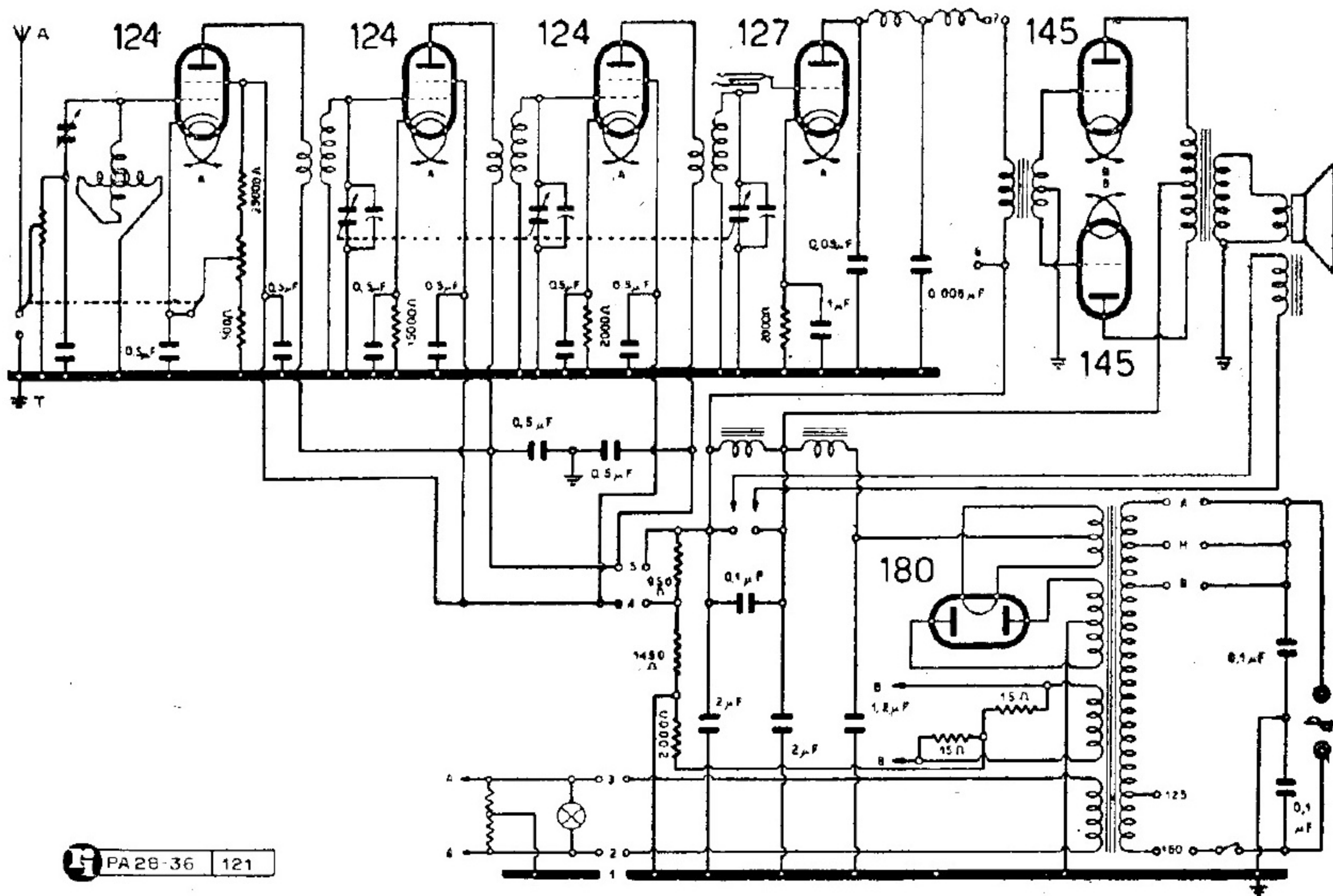
RADIOMARELLI - MOD. « MUSAGETE I »
