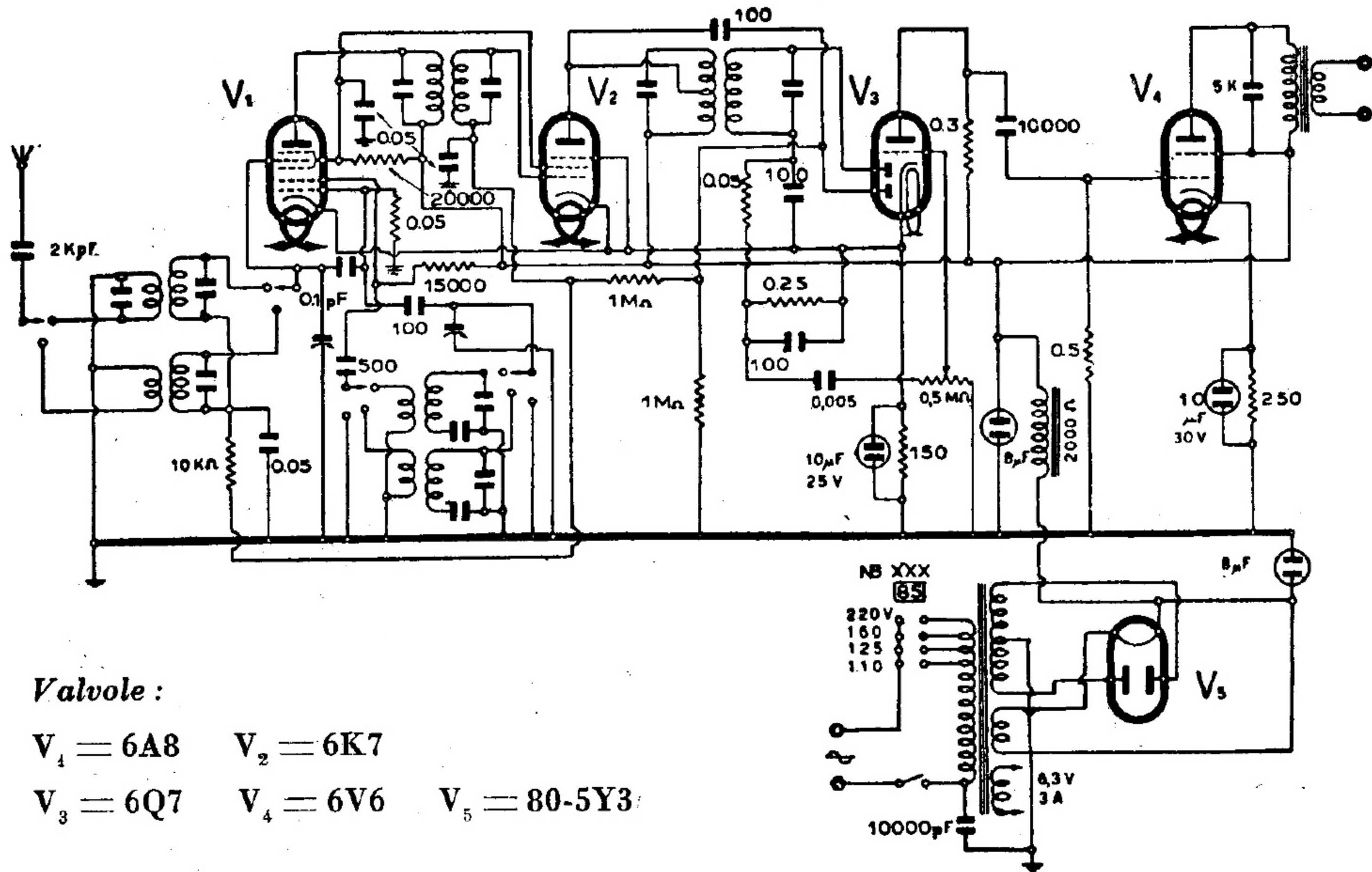
RADIO SAVOIA - MOD. « R 255. 1 »
