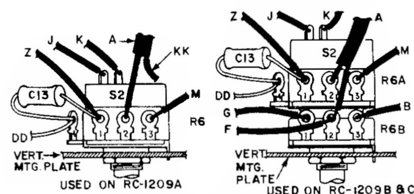
R6 & S2 Wiring
