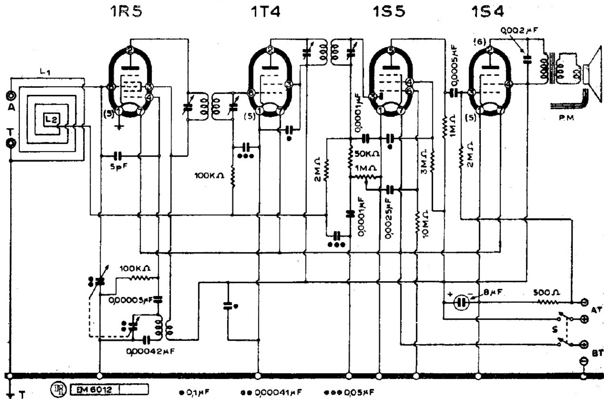
RCA VICTOR - MOD. « PERSONAL » I Serie
