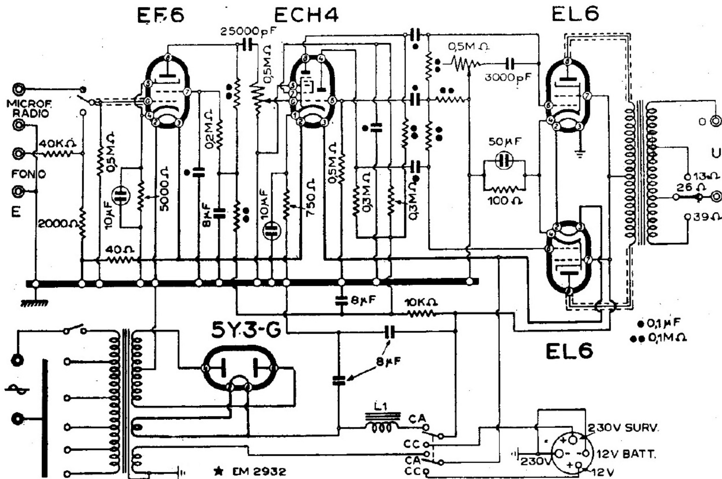
S.A.F.A.R. - AMPLIFICATORE 10 W MOD. « 509/A »
