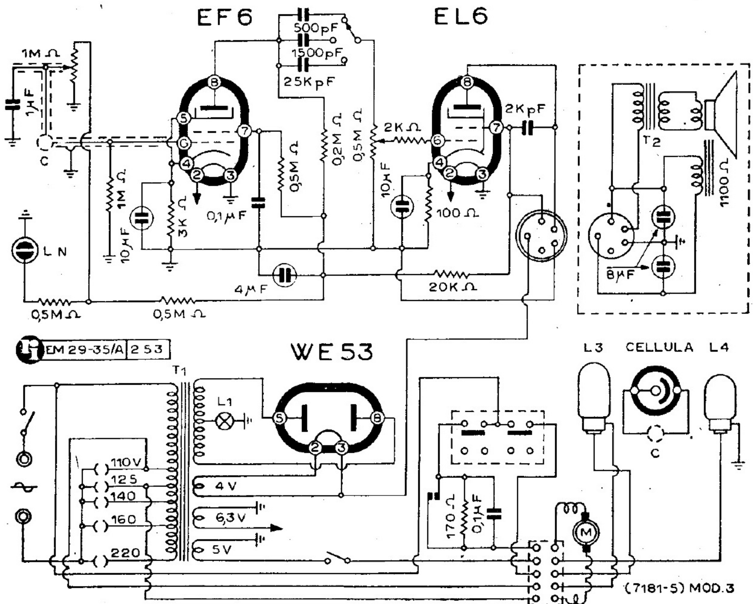
S.A.F.A.R. - AMPLIFICATORI MODD. « P.E.M. » I (sopra) e III Serie (sotto) PER PROIETTORE SONORO 16 mm (III serie per proiettori con numero di matricola dal 2338 in avanti)
