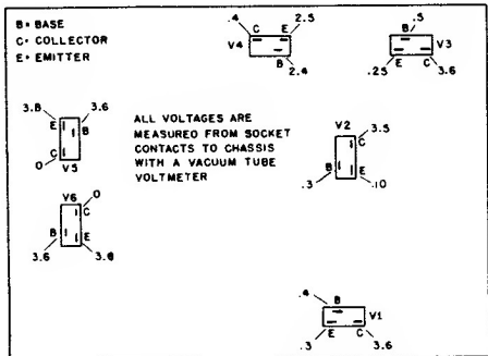
VOLTAGE TABLE
