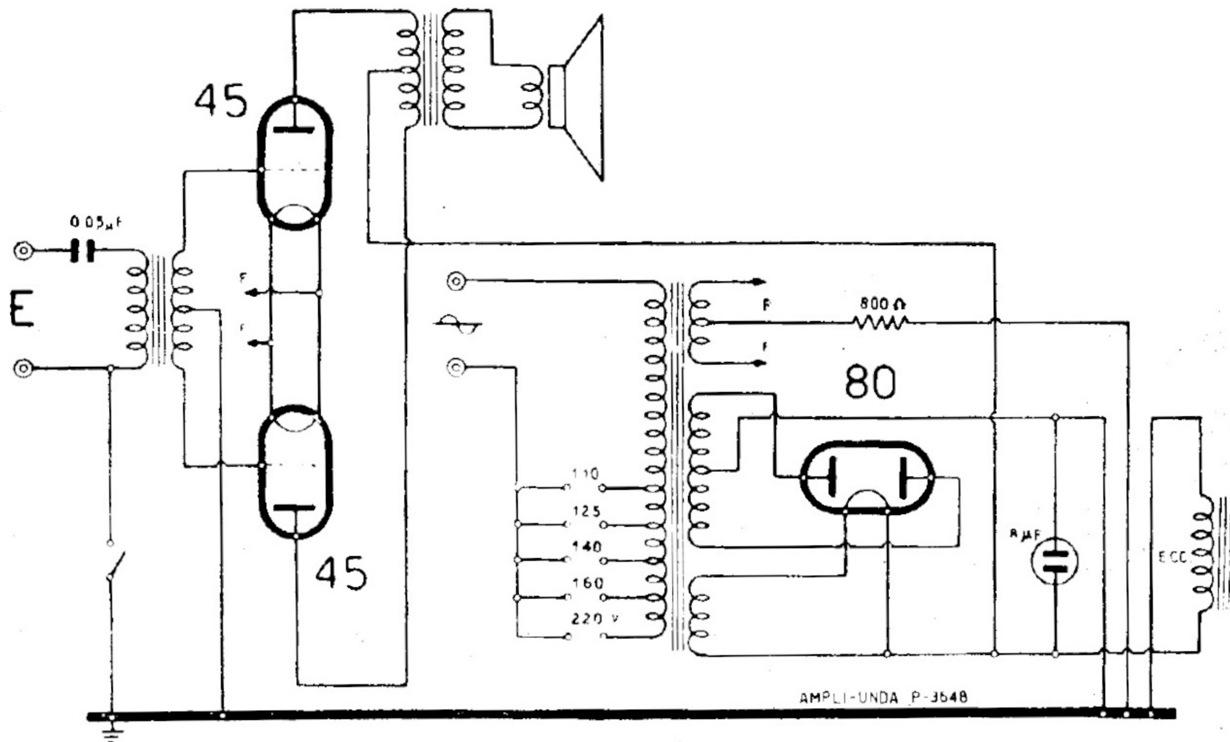
UNDA RADIO - AMPLIFICATORE MOD. « AMPLI UNDA »
