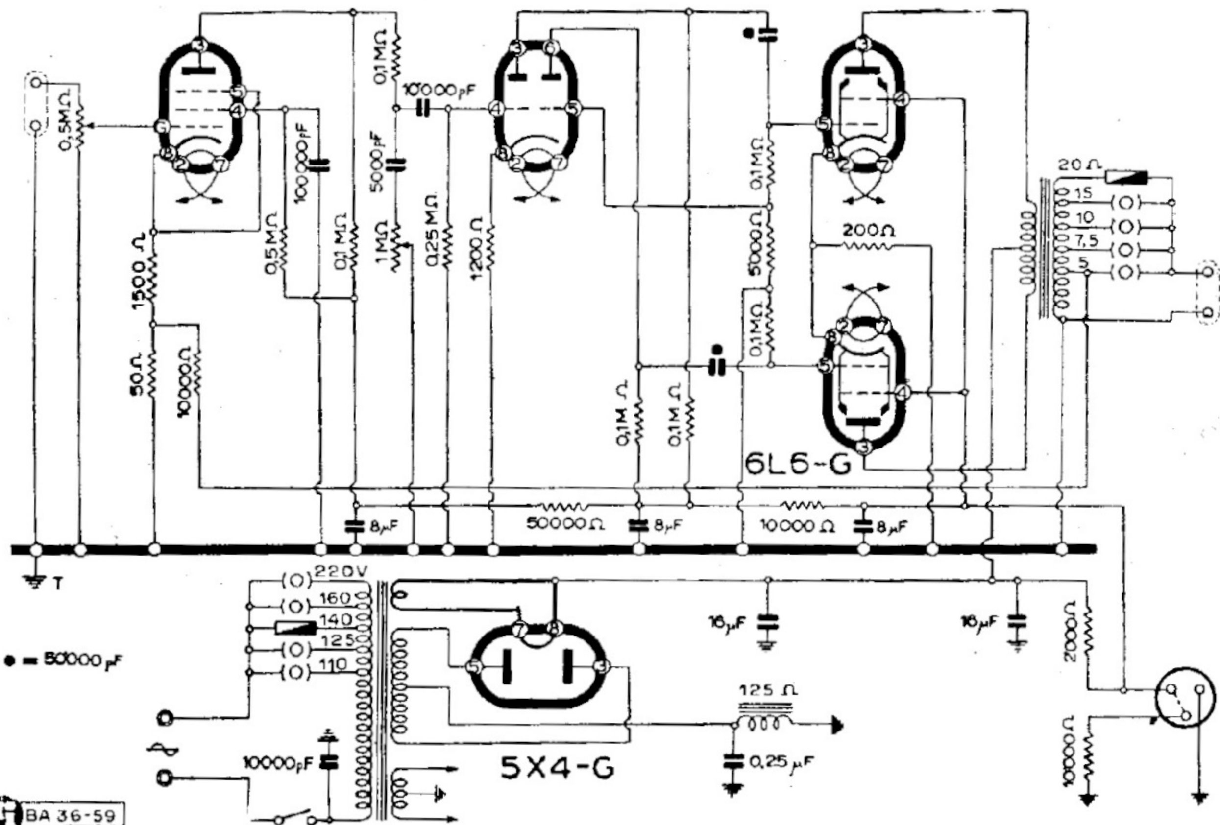
UNDA RADIO - AMPLIFICATORE FISSO MOD. « P5/1 »
