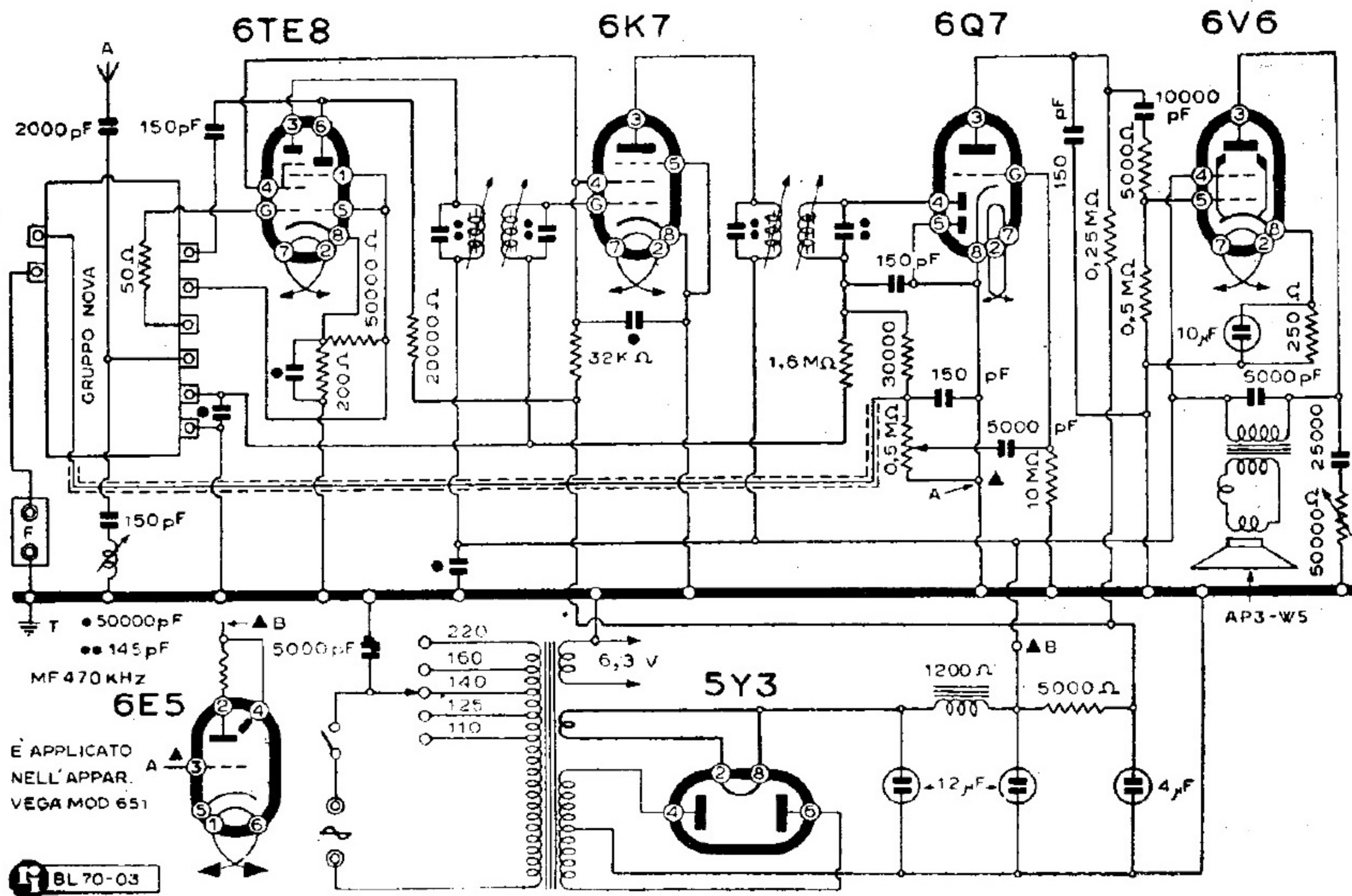
VEGA - B. P. RADIO MOD. « 551 »
