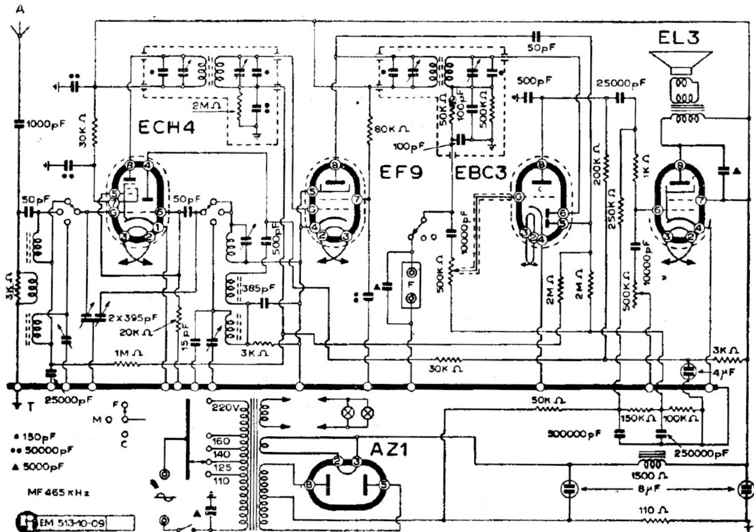
VIS RADIO - MOD. « TICINO »
