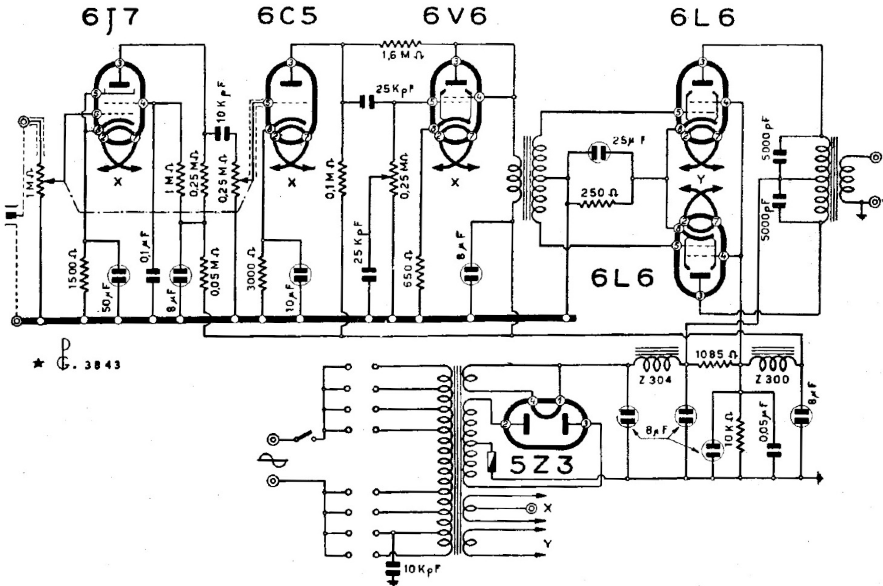
WATT RADIO - AMPLIFICATORE MOD. « 630 »
