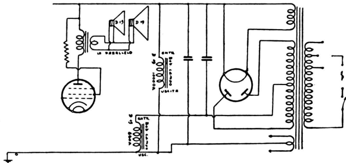
Modifica del sistema di eccitazione dei dinamici dei tipi « duofono » serie « Orfeo » e « 659 ».
