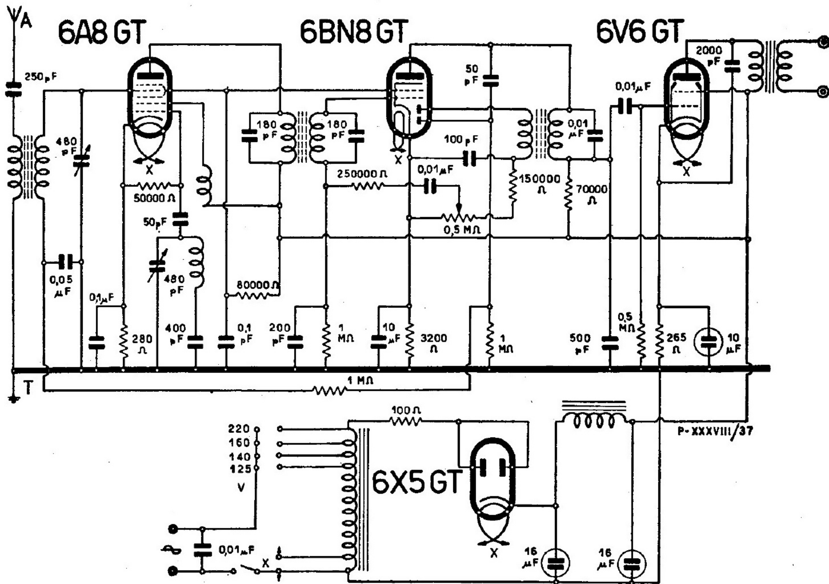
WATT RADIO : MOD. « CUCCIOLO »
