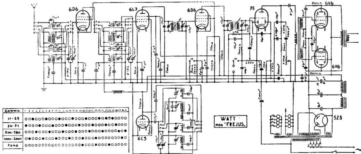
WATT RADIO. — Modello Frejus e Frejus Fono. — Produzione 1938-39. — Gamme: cc. (13-25), c. (25-50), m. (200-580), l. (1100-2000). — Media frequenza: 485 kHz
