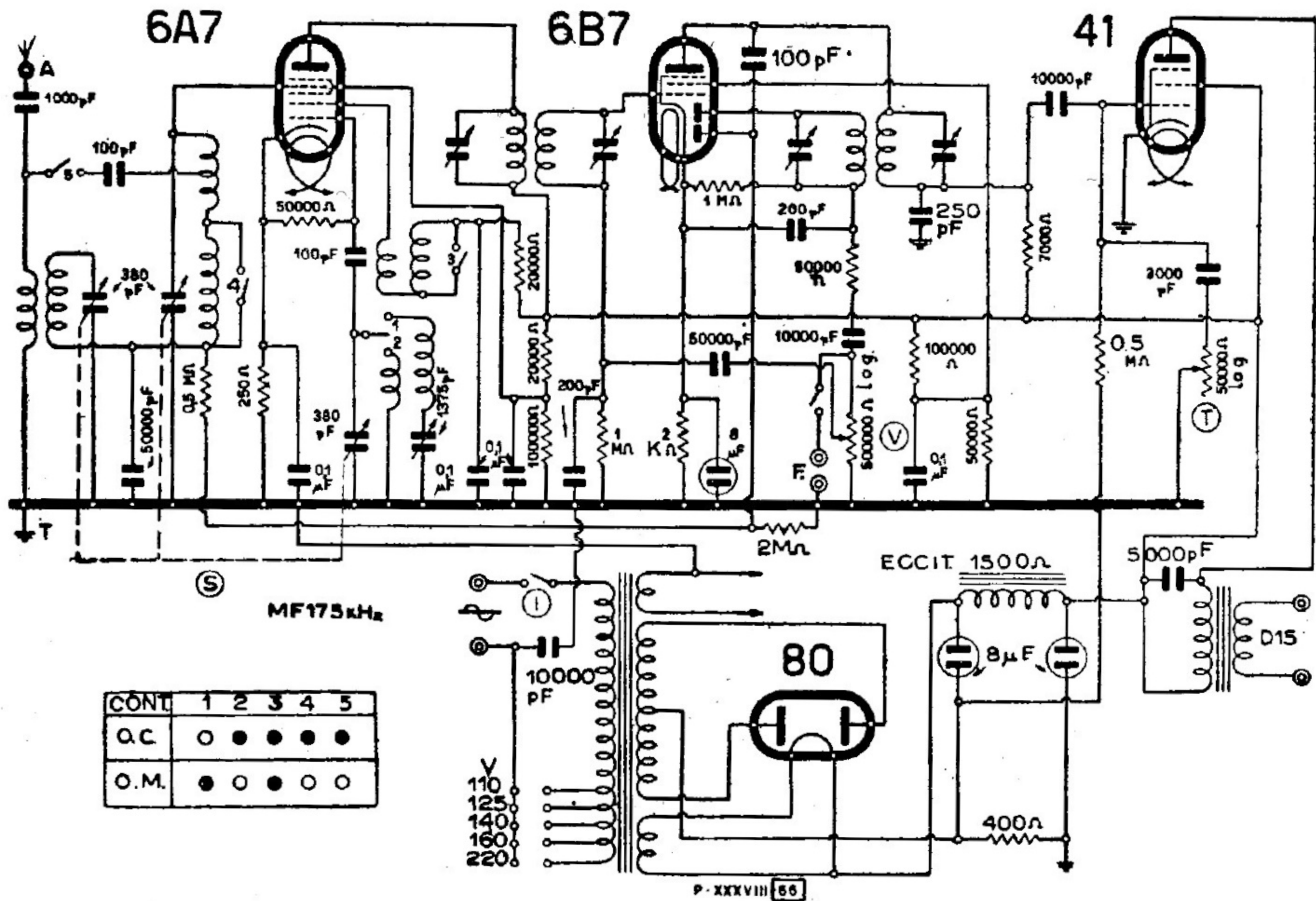
WATT RADIO - MOD. « ONDINA IV »
