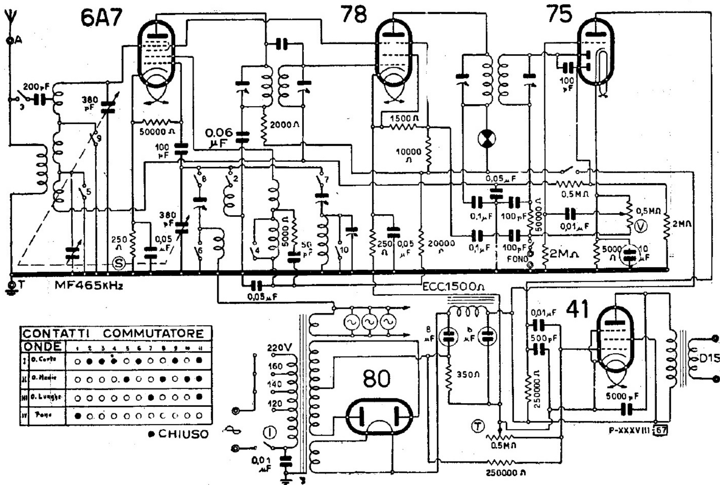
WATT RADIO - MOD. «SIDERODINA»
