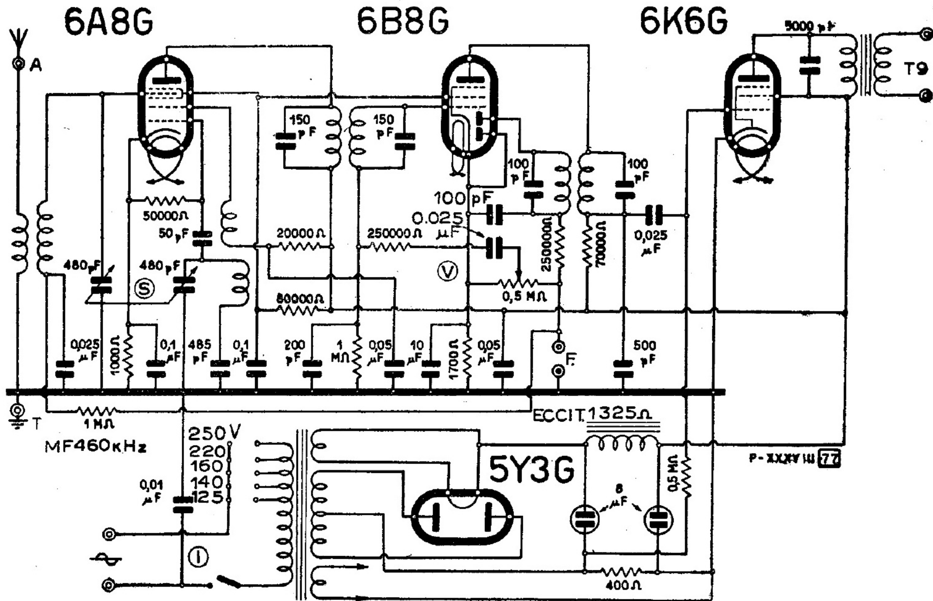
WATT RADIO - MOD. «STELLA»
