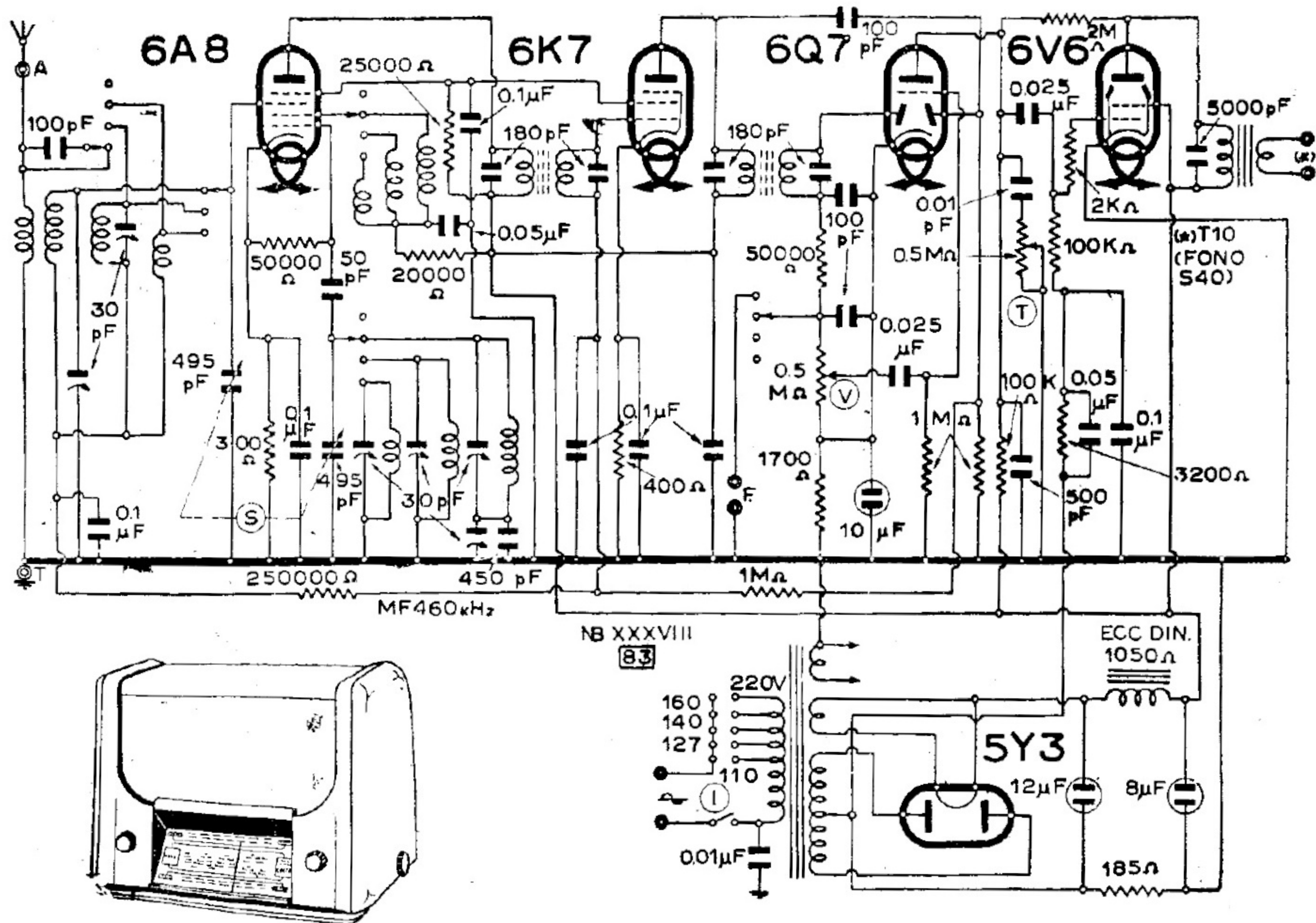
WATT RADIO - MOD. « SUPER STELLA 42 »
