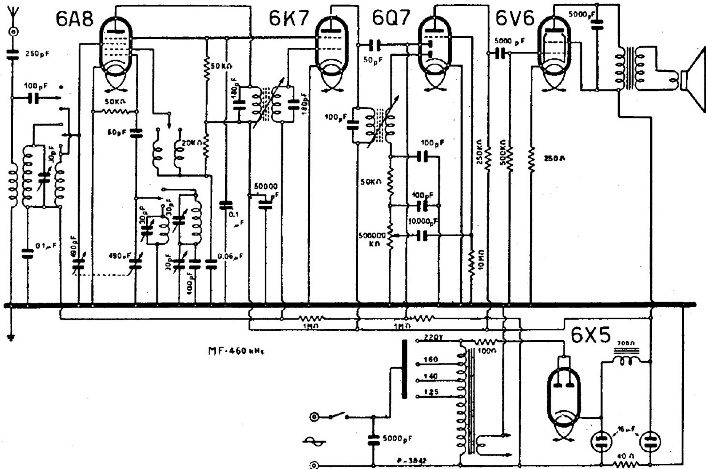
WATT RADIO - MOD. « TESORO II »
